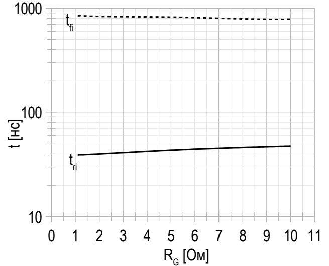
Рисунок 14 – типичное время переключения от сопротивления в затворе, FRD.
