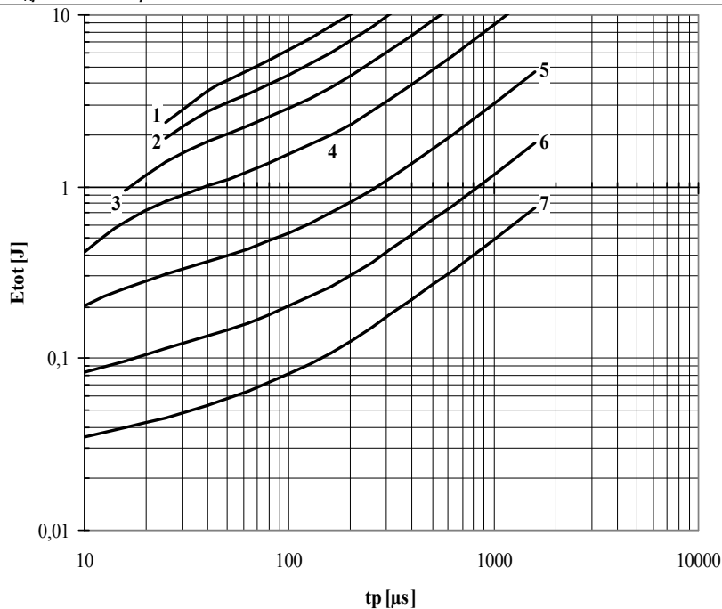
Рис. 25 – Зависимость энергии потерь за один синусоидальный импульс тока от длительности импульса
