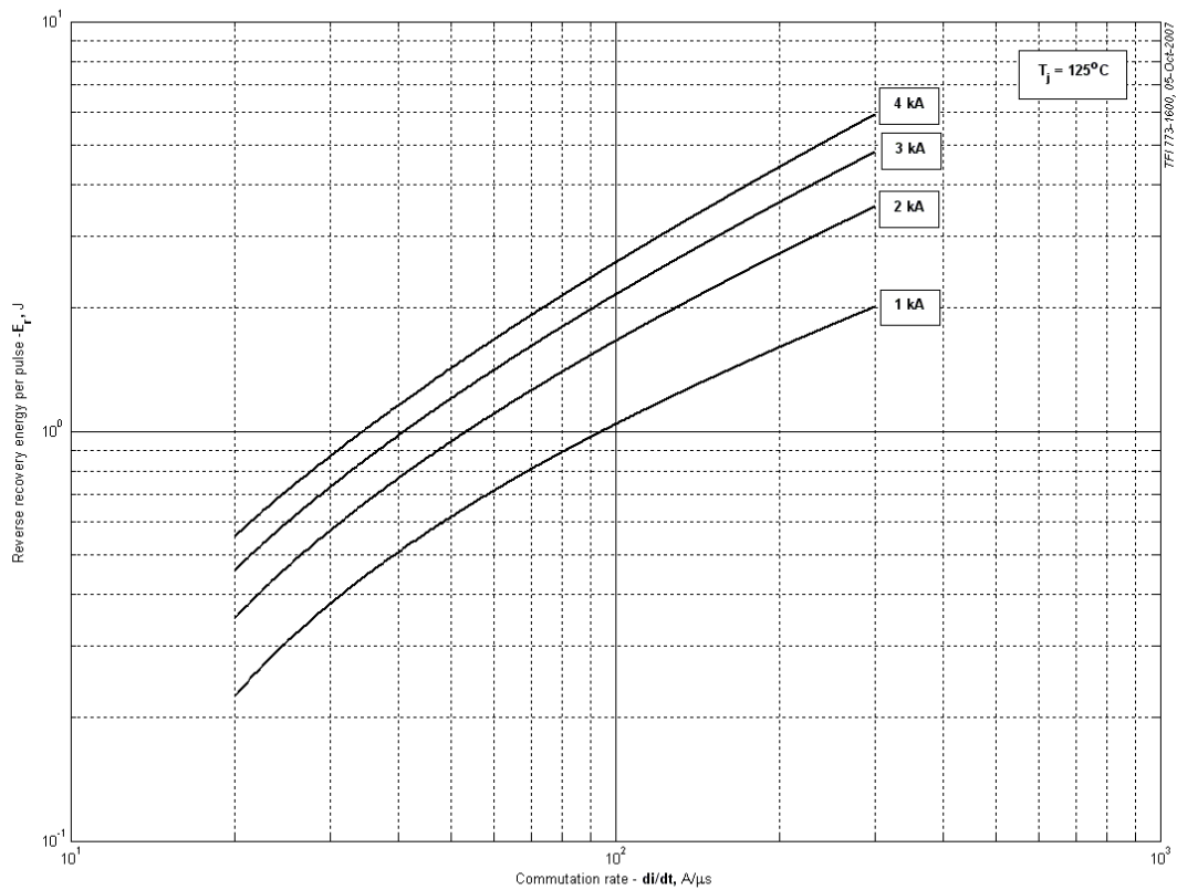
Рис. 7 – Энергия обратного восстановления за импульс
