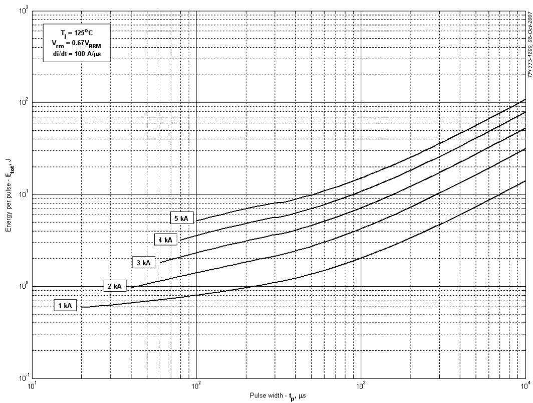
Рис. 24 – Суммарная энергия потерь одного прямоугольного импульса тока
