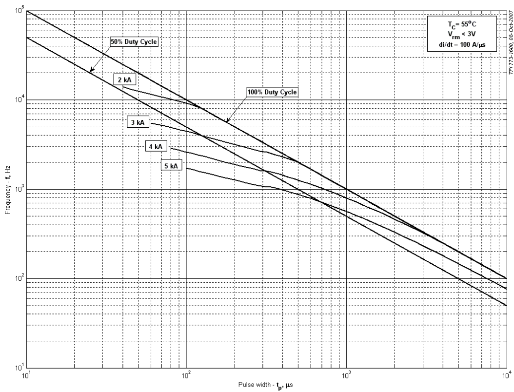
Рис. 14 – Зависимость частоты прямоугольных импульсов тока от длительности импульсов
