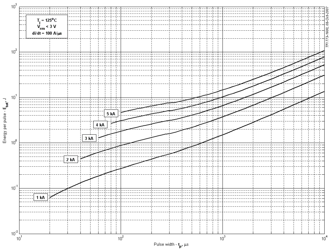
Рис. 18 – Суммарная энергия потерь одного прямоугольного импульса тока
