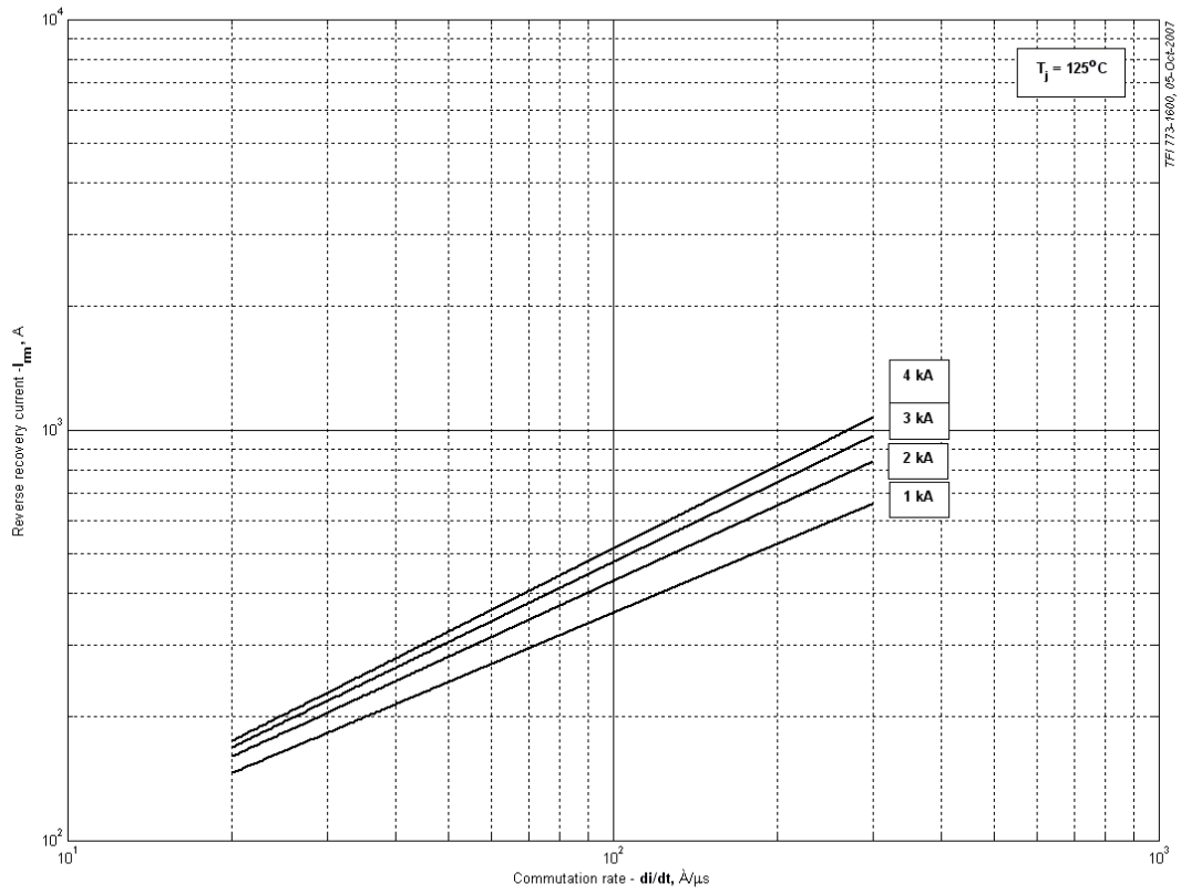
Рис. 5 – Максимальный обратный ток восстановления, I_{rr}
