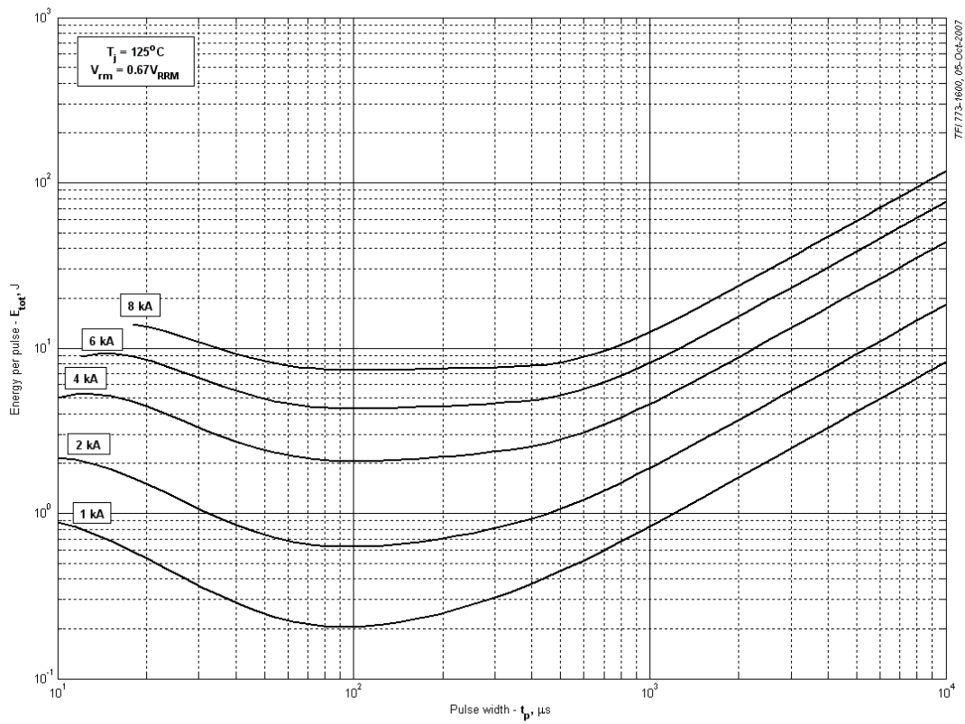
Рис. 9 – Суммарная энергия потерь одного синусоидального импульса тока
