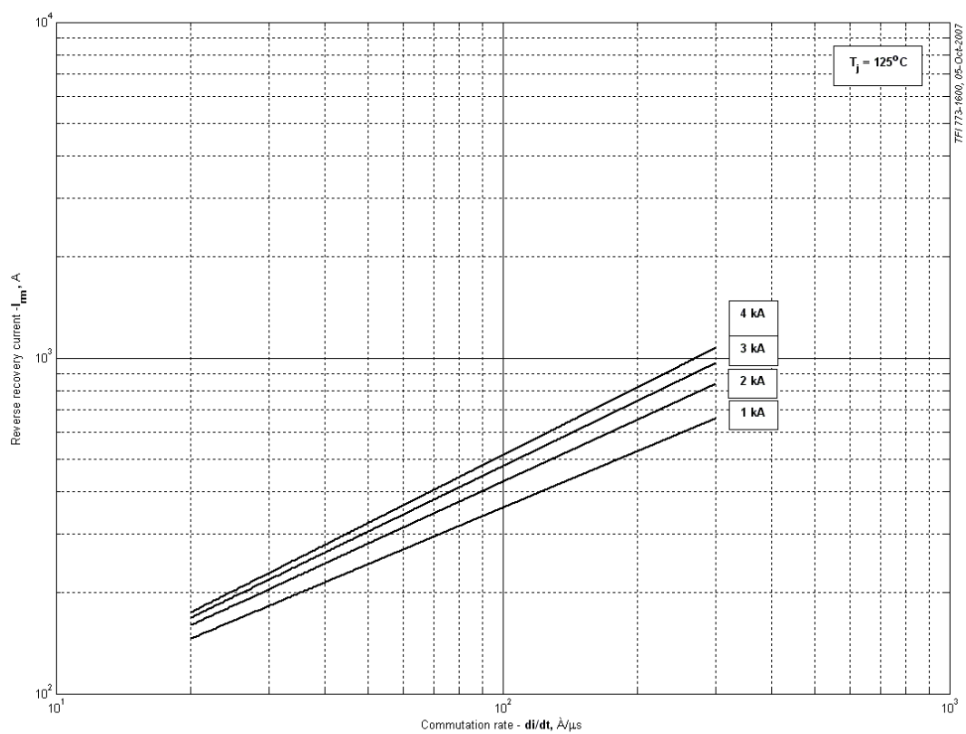
Рис. 5 – Максимальный ток обратного восстановления, I_{rrm}
