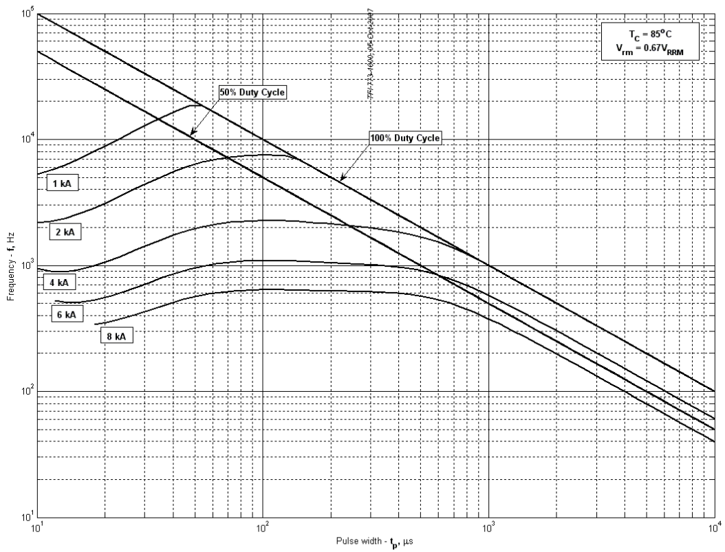
Рис. 13 – Зависимость частоты синусоидальных импульсов тока от длительности импульсов
