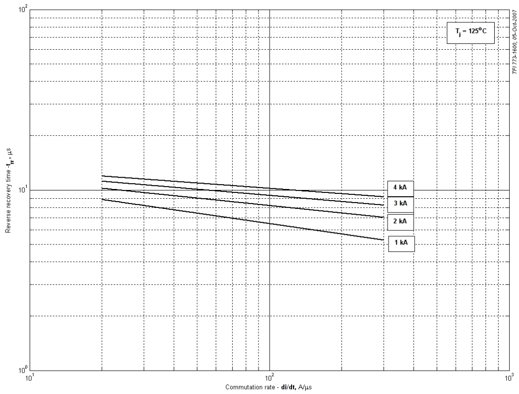
Рис. 6 – Максимальное время обратного восстановления, t_{rr} (по ГОСТ 24461, хорда 50%)
