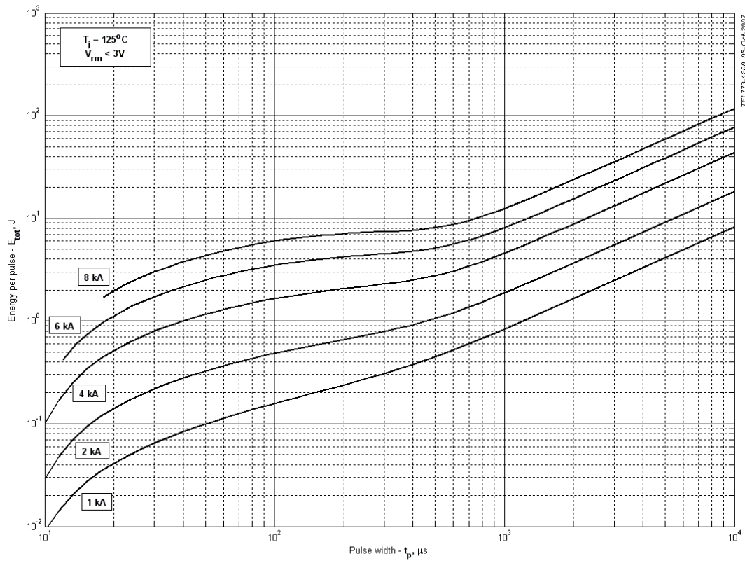
Рис. 8 – Суммарная энергия потерь одного синусоидального импульса тока
