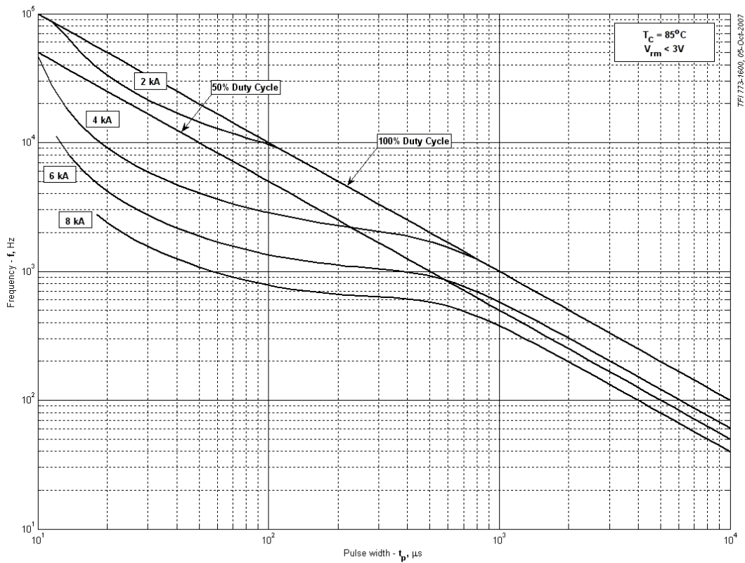
Рис. 11 – Зависимость частоты синусоидальных импульсов тока от длительности импульсов
