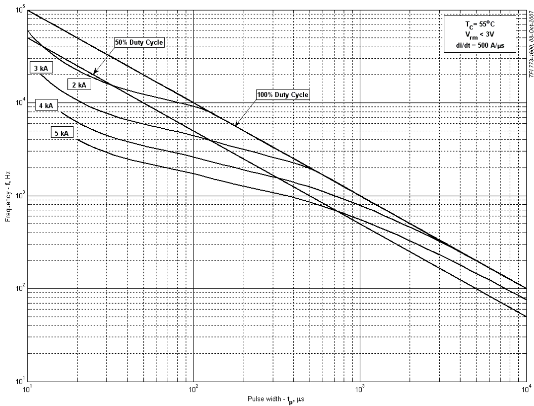
Рис. 15– Зависимость частоты прямоугольных импульсов тока от длительности импульсов
