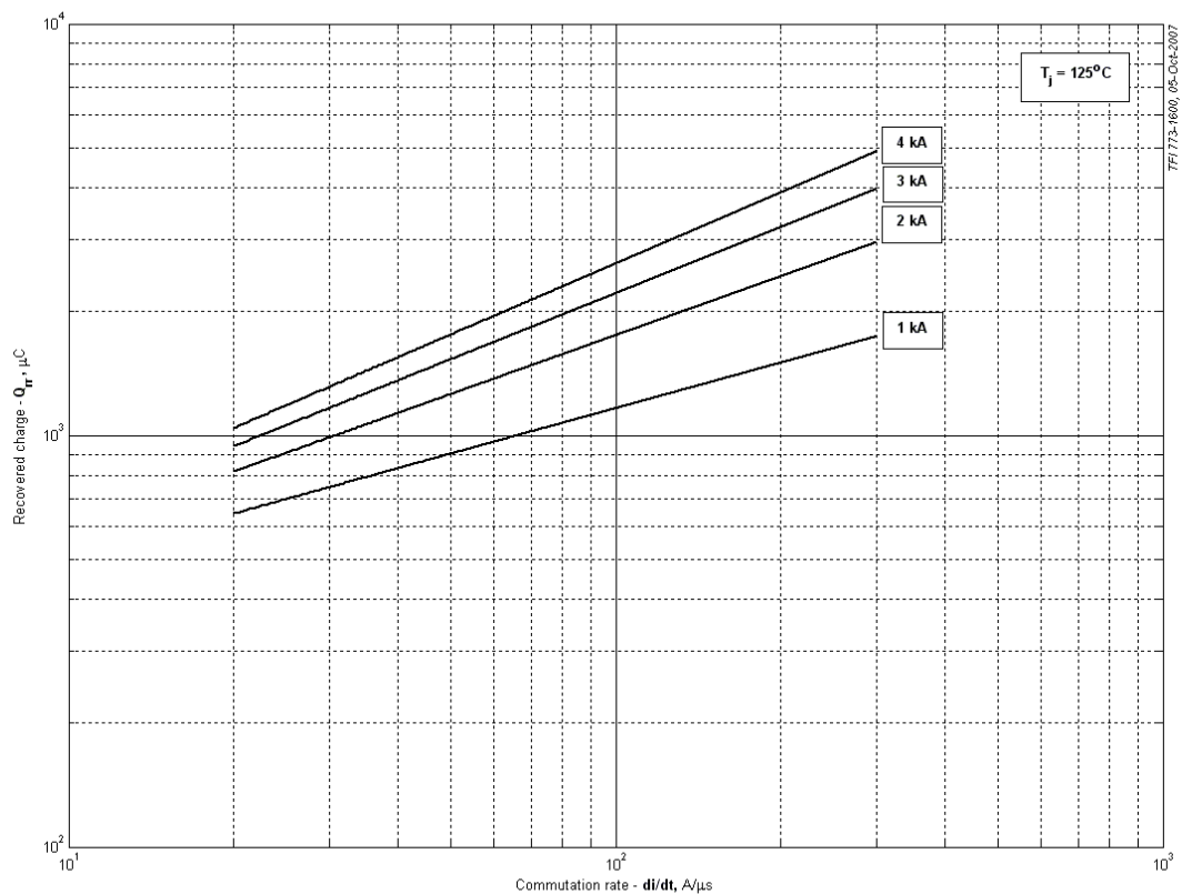
Рис. 4 – Максимальный заряд обратного восстановления, Q_{rr} (по ГОСТ 24461, хорда 50%)
