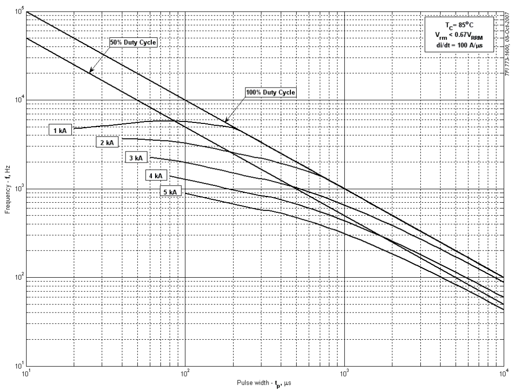
Рис. 22 – Зависимость частоты прямоугольных импульсов тока от длительности импульсов
