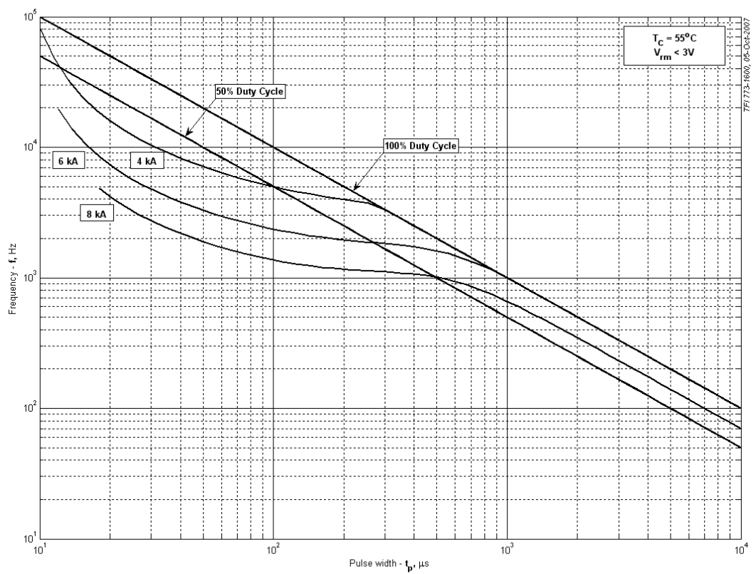
Рис. 10 – Зависимость частоты синусоидальных импульсов тока от длительности импульсов
