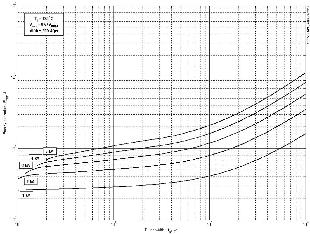
Рис. 25 – Суммарная энергия потерь одного прямоугольного импульса тока
