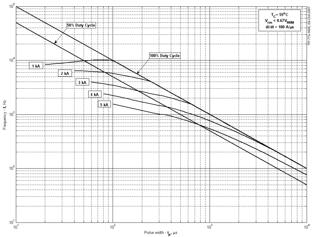
Рис. 20 – Зависимость частоты прямоугольных импульсов тока от длительности импульсов
