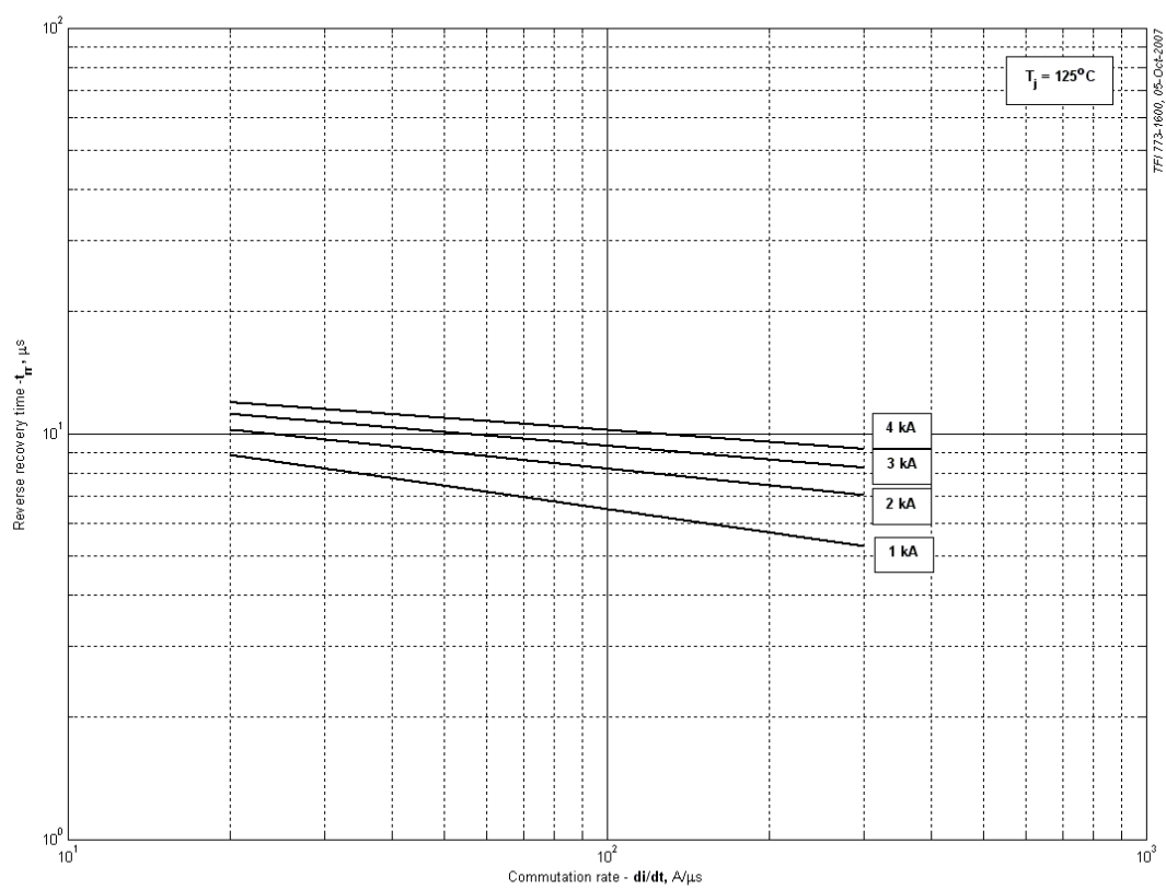
Рис. 6 – Максимальное время обратного восстановления, t_{rr} (по ГОСТ 24461, хорда 50%)
