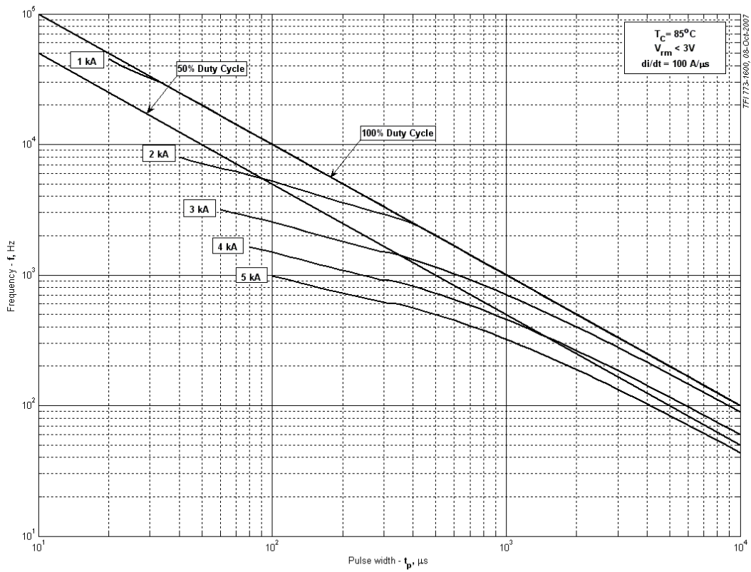
Рис. 17 – Зависимость частоты прямоугольных импульсов тока от длительности импульсов
