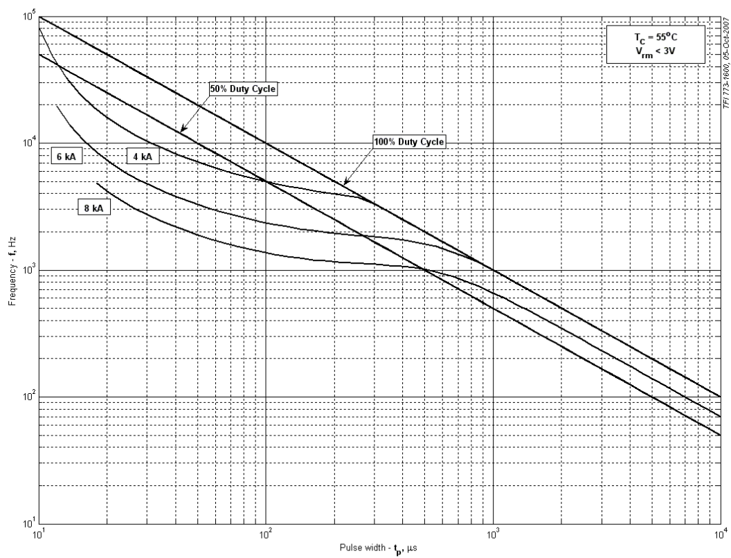
Рис. 10 – Зависимость частоты синусоидальных импульсов тока от длительности импульсов
