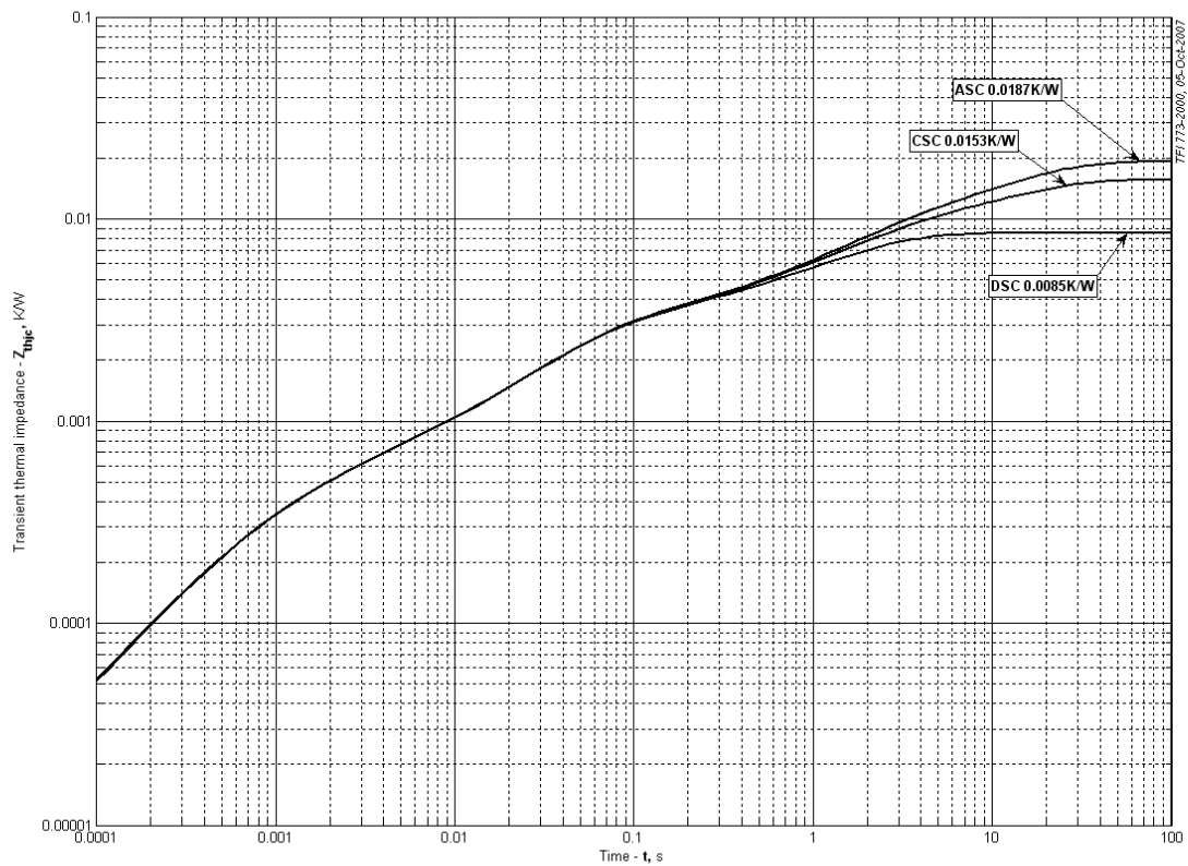
Рис. 2 – Переходное тепловое сопротивление
