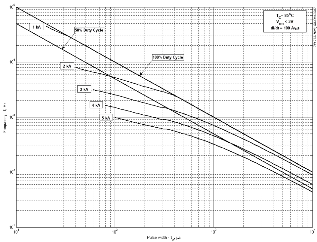
Рис. 16 – Зависимость частоты прямоугольных импульсов тока от длительности импульсов
