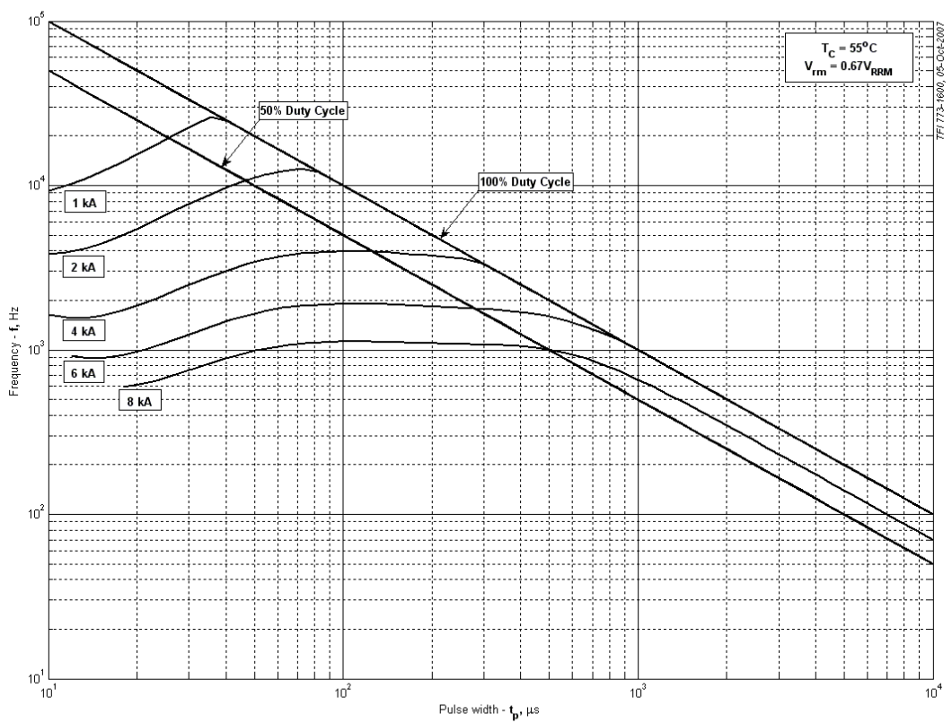
Рис. 12 – Зависимость частоты синусоидальных импульсов тока от длительности импульсов
