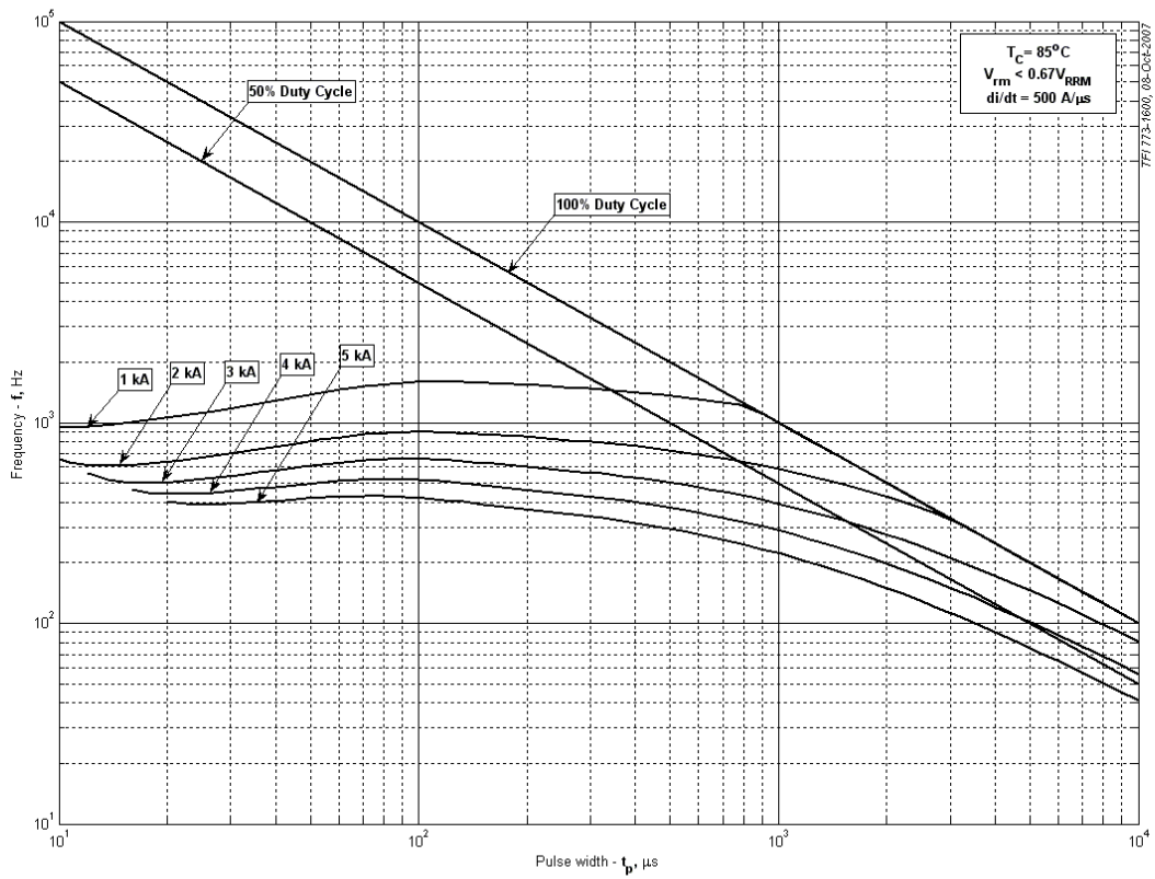
Рис. 23 – Зависимость частоты прямоугольных импульсов тока от длительности импульсов
