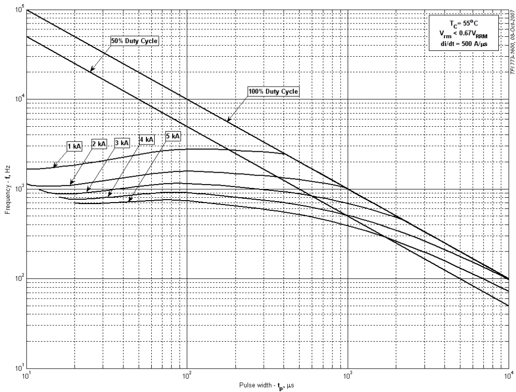
Рис. 21 – Зависимость частоты прямоугольных импульсов тока от длительности импульсов
