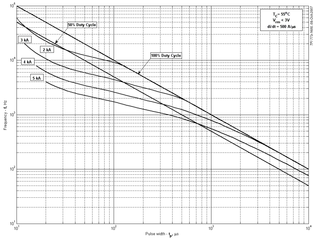
Рис. 15– Зависимость частоты прямоугольных импульсов тока от длительности импульсов
