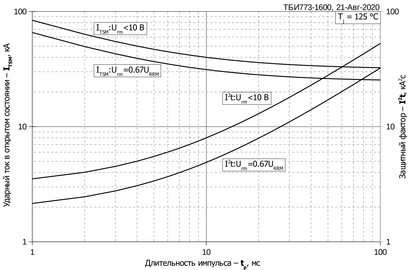
Рис. 26 – Максимальные ударные и I^2t характеристики
