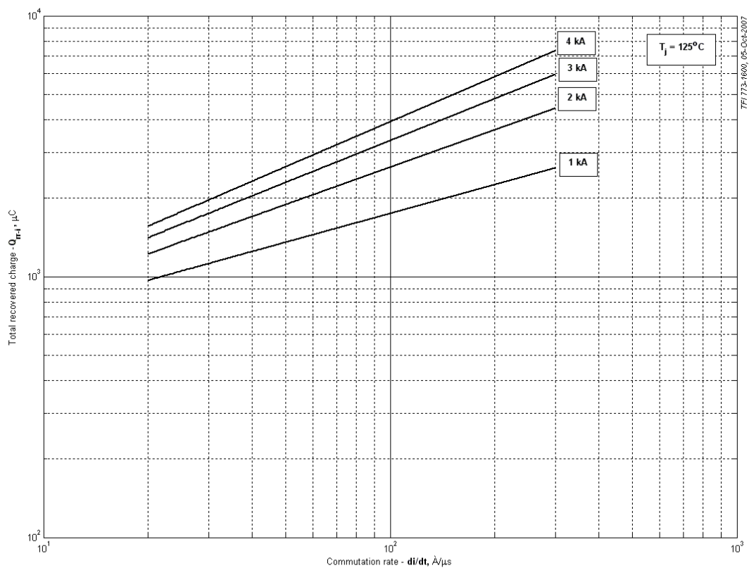
Рис. 3 – Максимальный интегральный заряд обратного восстановления, Q_{rr-i}
