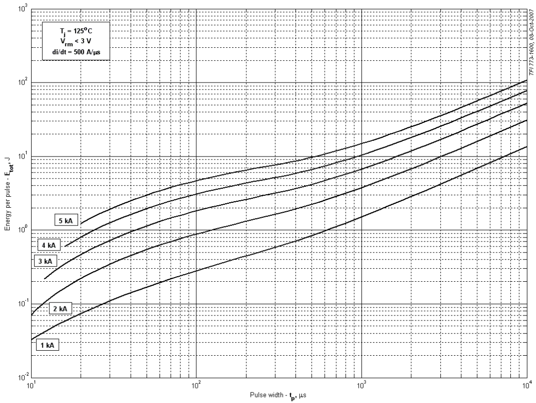
Рис. 19 – Суммарная энергия потерь одного прямоугольного импульса тока
