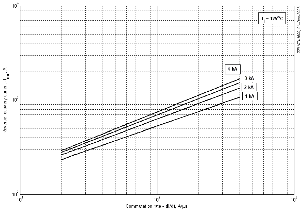
Рис. 5 – Максимальный обратный ток восстановления, I_{rr}
