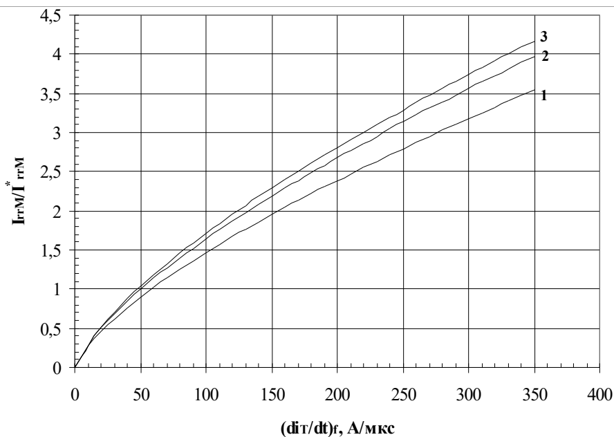
Рис. 33 – Максимальная зависимость обратного тока восстановления I_{rr} от скорости спада 1 - I_T = 0,5 I_{TAV} ; 2 - I_T = I_{TAV} ; 3 - I_T = 1,5 I_{TAV} .
