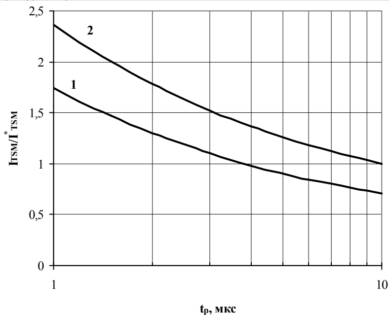
Рис. 22 – Зависимость ударного тока I_{TSM} от длительности импульса t_p для начальной температуры перехода: 1 – T_j=125\text{ }^\circ\text{C} 2 – T_j=25\text{ }^\circ\text{C}
