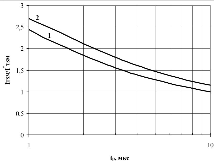
Рис. 21 – Зависимость ударного тока I_{TSM} от длительности импульса t_p для полусинусоидального импульса. 1 – T_j=125\text{ }^\circ\text{C} 2 – T_j=25\text{ }^\circ\text{C}
