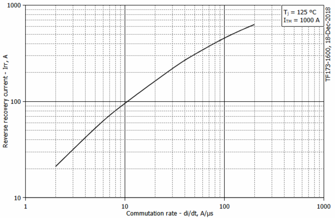
Рис. 5 – Максимальный обратный ток восстановления, I_{rr}
