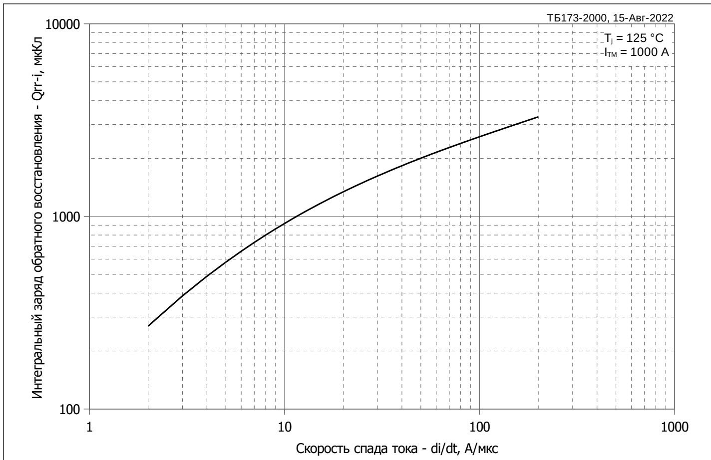
Рис. 5 – Зависимость максимального интегрального заряда обратного восстановления Q_{rr-i} от скорости спада тока di/dt в открытом состоянии
