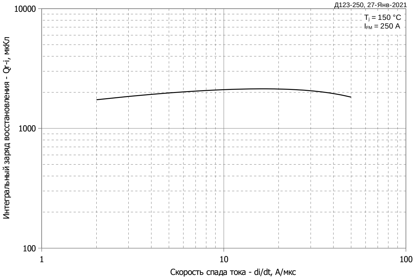
Рис. 3 – Зависимость заряда восстановления Q_{r-i} (интегральный) от скорости спада прямого тока di_R/dt
