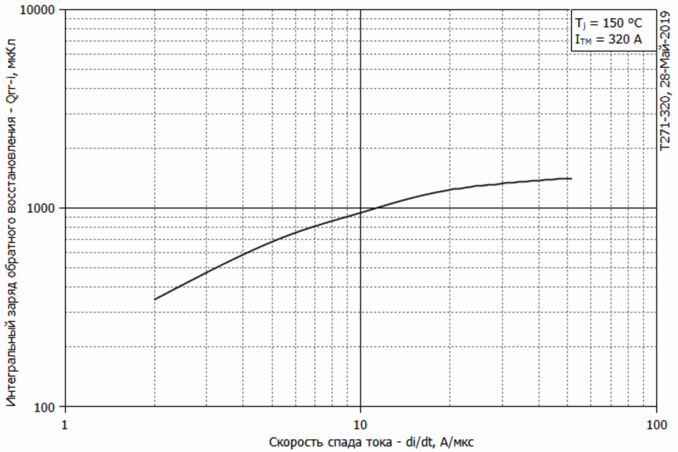
Рис. 3 – Зависимость максимального интегрального заряда обратного восстановления Q rr-и от скорости спада тока di R /dt в открытом состоянии
