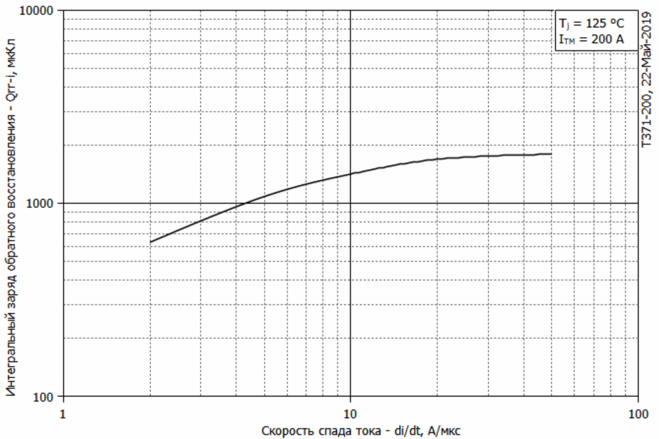
Рис. 3 – Зависимость максимального интегрального заряда обратного восстановления Q rr от скорости спада тока di R /dt в открытом состоянии
