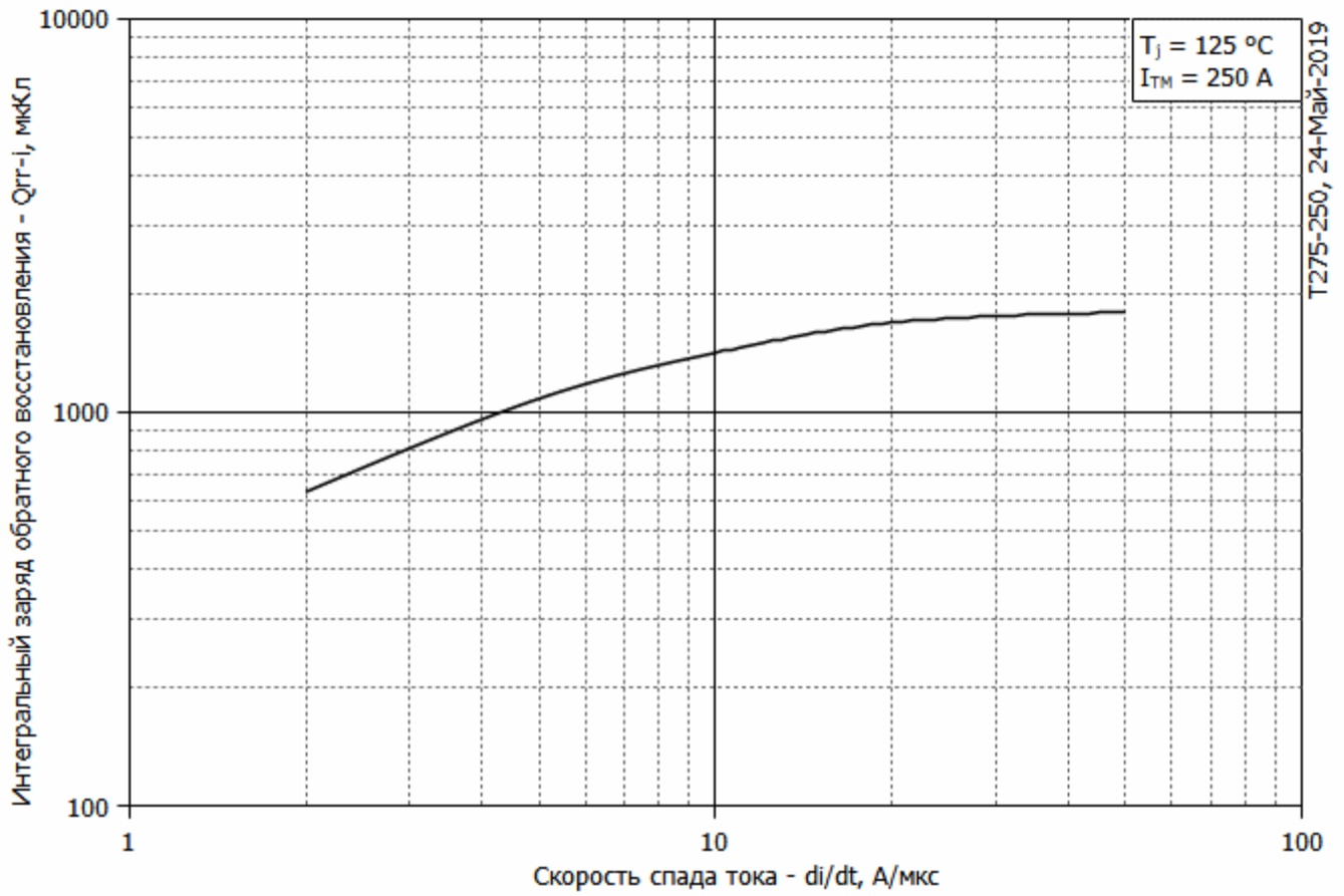
Рис. 3 – Зависимость максимального интегрального заряда обратного восстановления Q гр-и от скорости спада тока di R /dt в открытом состоянии
