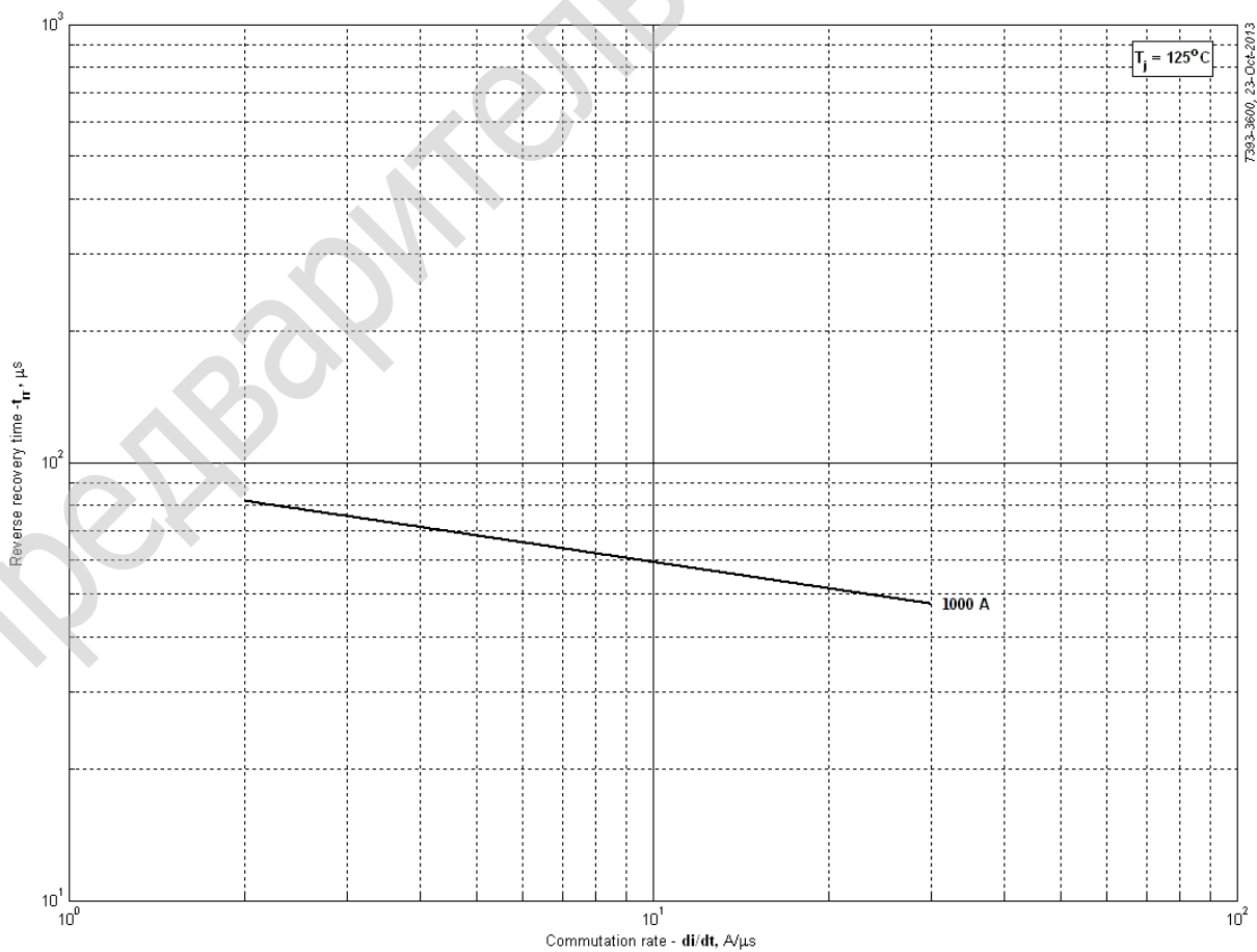
Рис. 8 - Зависимость максимального времени обратного восстановления t_{гр} от скорости спада тока di_R/dt (по ГОСТ 24461, хорда 25%) в открытом состоянии
