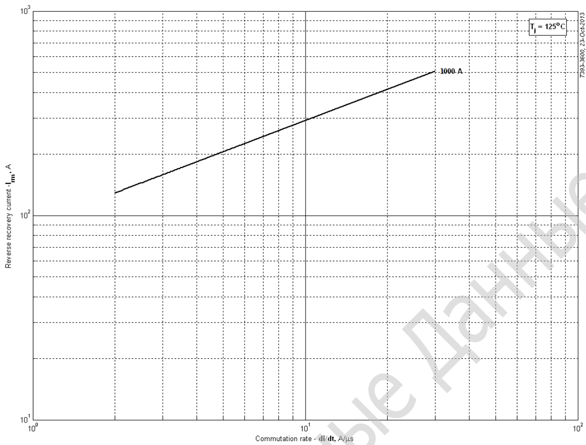
Рис. 7 – Зависимость максимального обратного тока восстановления I_{гр} от скорости спада тока di_R/dt в открытом состоянии
