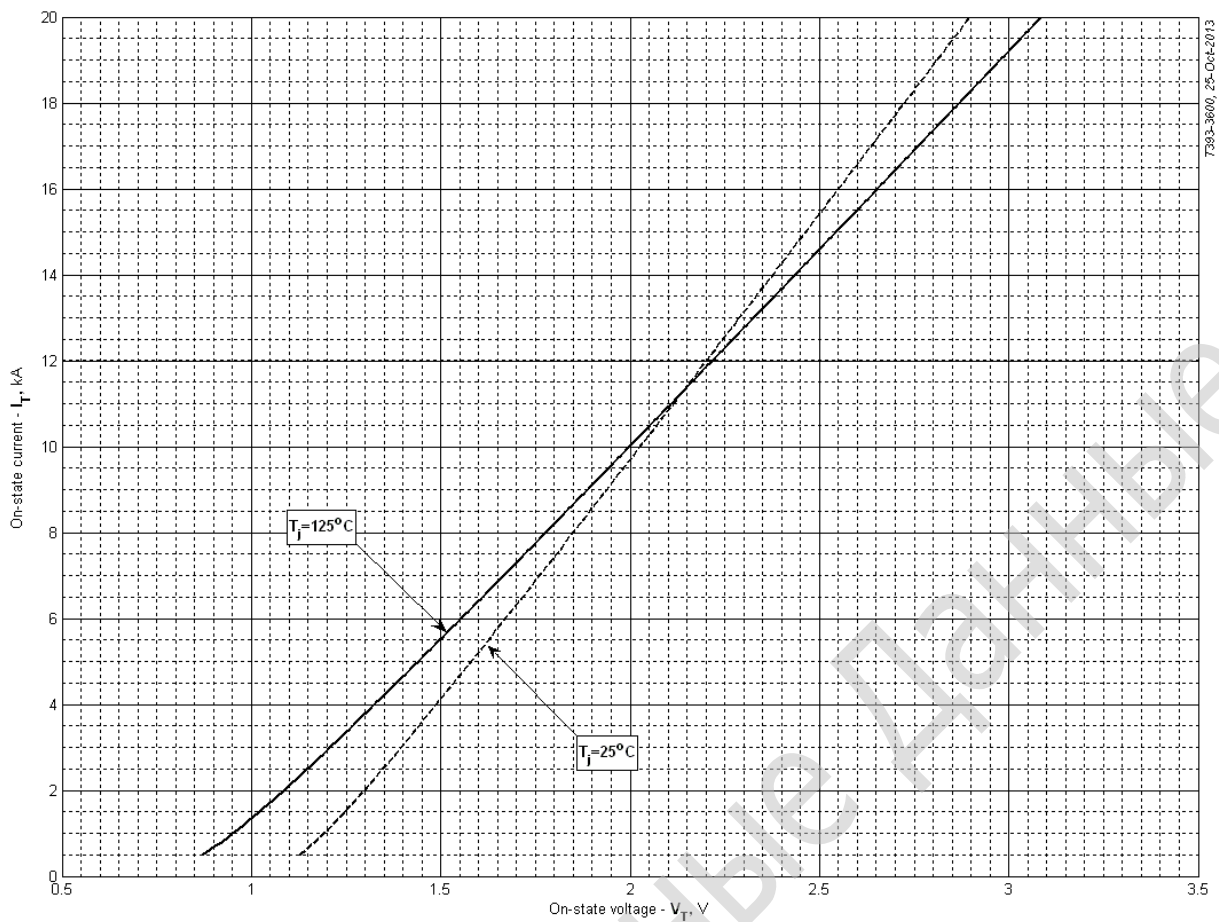
Рис. 1 – Предельная вольт – амперная характеристика
