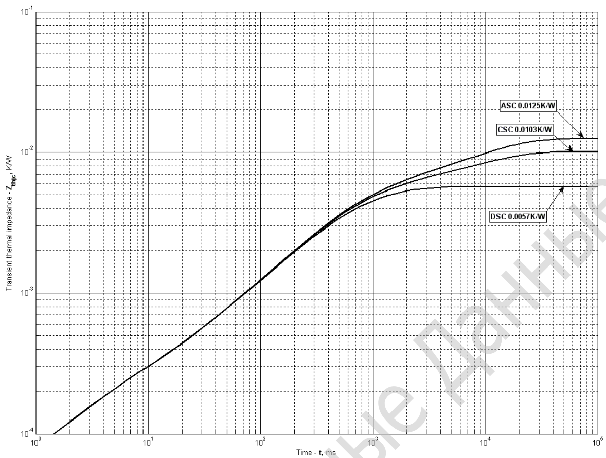
Рис. 2 – Зависимость переходного теплового сопротивления Z_{thjc} от времени t Аналитическая зависимость переходного теплового сопротивления переход — корпус:
