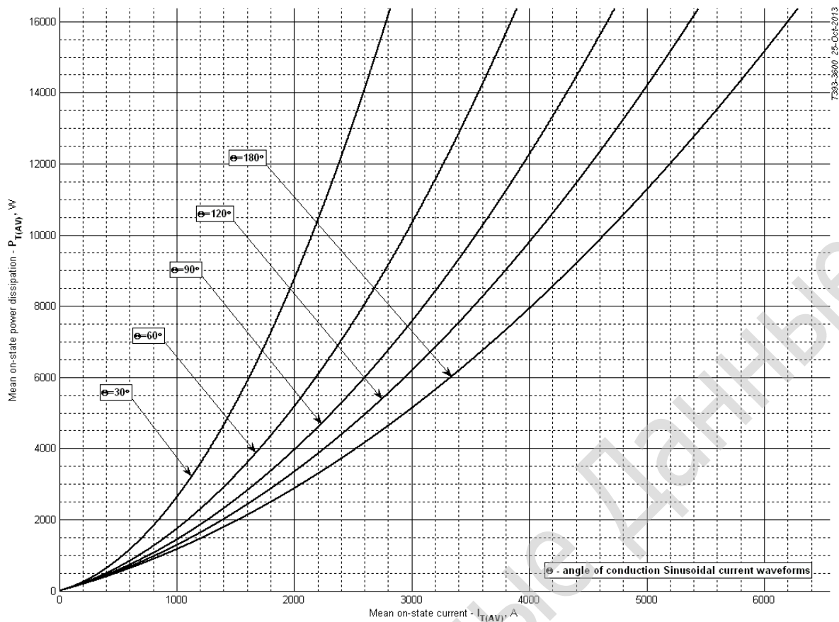
Рис. 9 - Зависимость потерь мощности P_{TAV} от среднего тока в открытом состоянии I_{TAV} синусоидальной формы при различных углах проводимости ( f=50 Гц)
