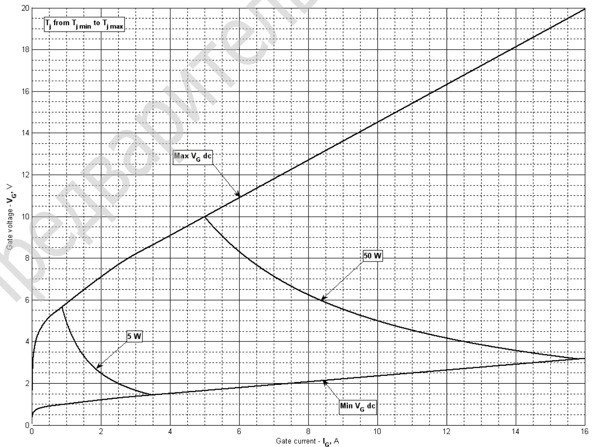
Рис. 4 – Вольт – амперная характеристика цепи управления – Кривые мощности
