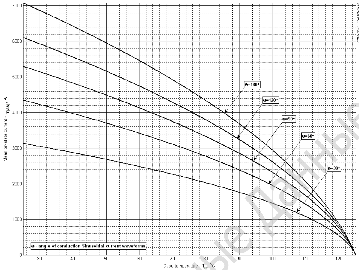
Рис. 11 – Зависимость среднего тока в открытом состоянии I_{TAV} от температуры корпуса T_c для синусоидальной формы тока при различных углах проводимости ( f=50 Гц)
