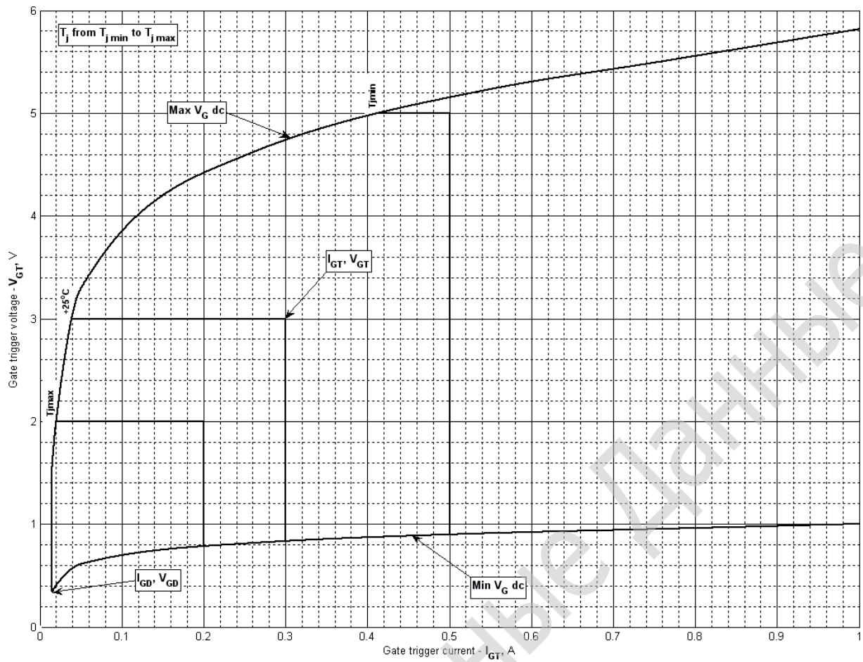
Рис. 3 – Вольт – амперная характеристика цепи управления
