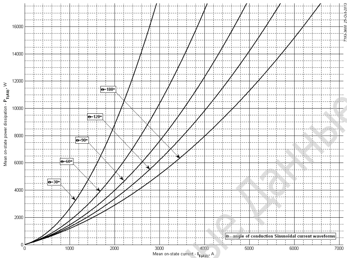
Рис. 9 - Зависимость потерь мощности P_{TAV} от среднего тока в открытом состоянии I_{TAV} синусоидальной формы при различных углах проводимости ( f=50 Гц, двухстороннее охлаждение)
