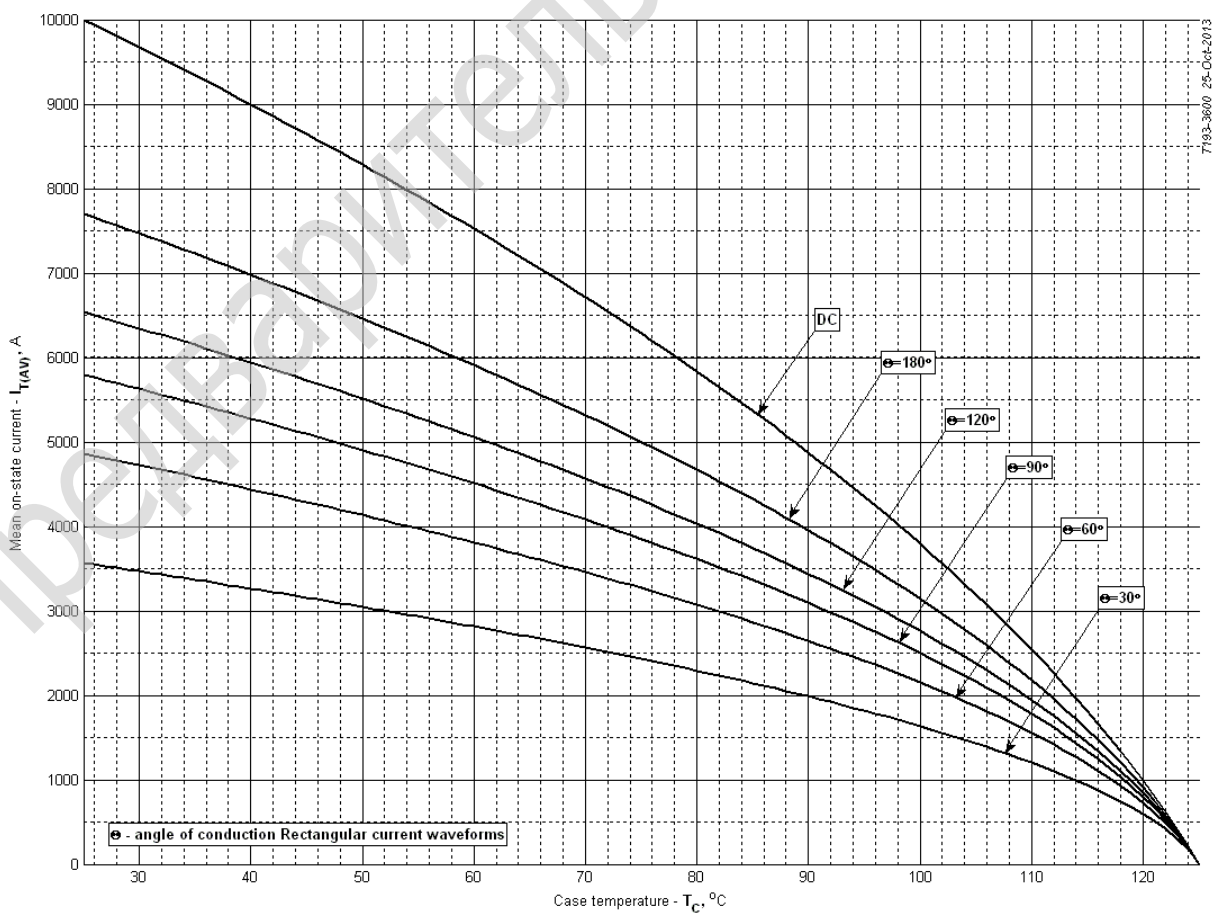
Рис. 12 - Зависимость среднего тока в открытом состоянии I_{TAV} от температуры корпуса T_c для прямоугольной формы тока при различных углах проводимости ( f=50 Гц)
