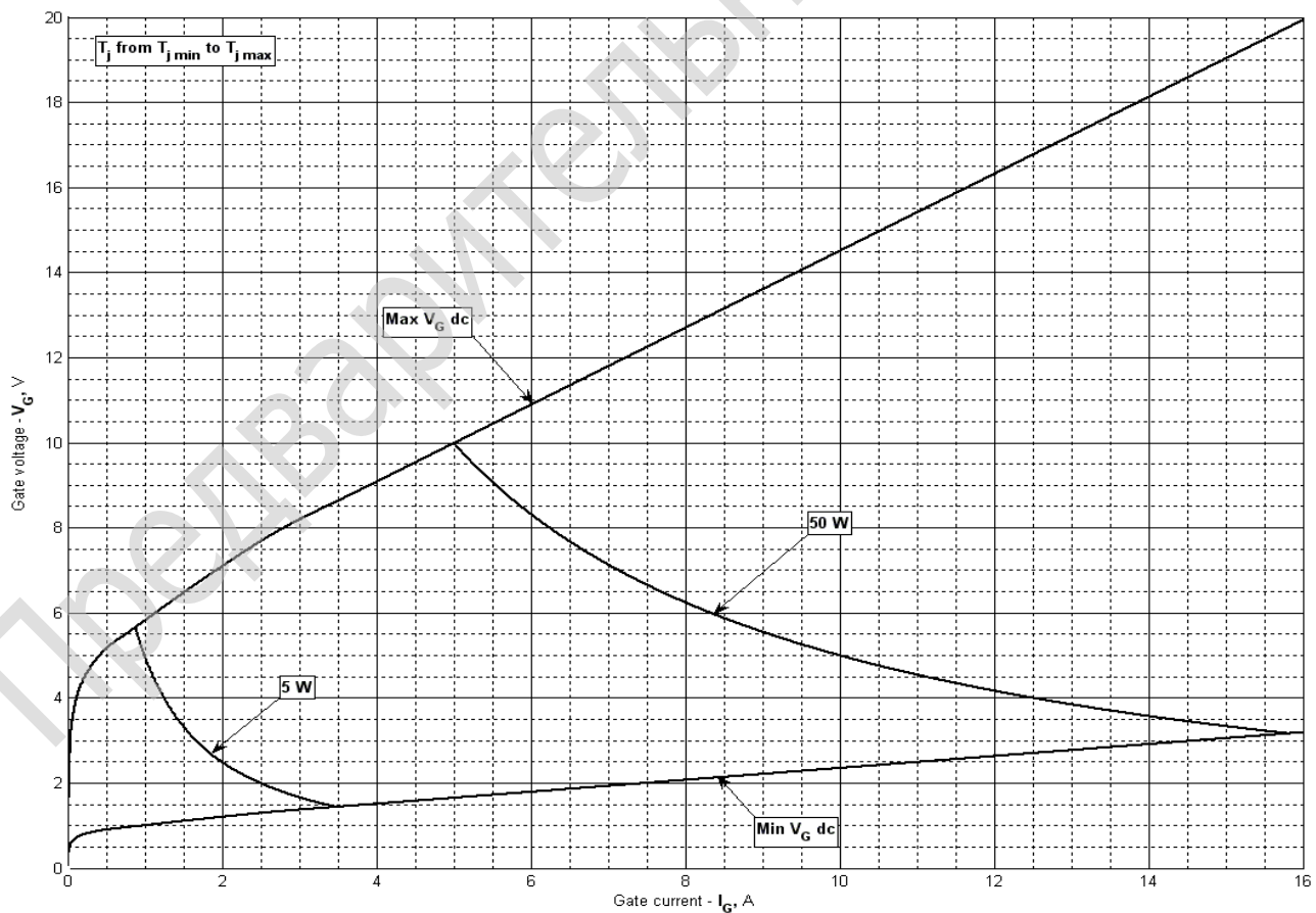
Рис. 4 – Вольт – амперная характеристика цепи управления – Кривые мощности
