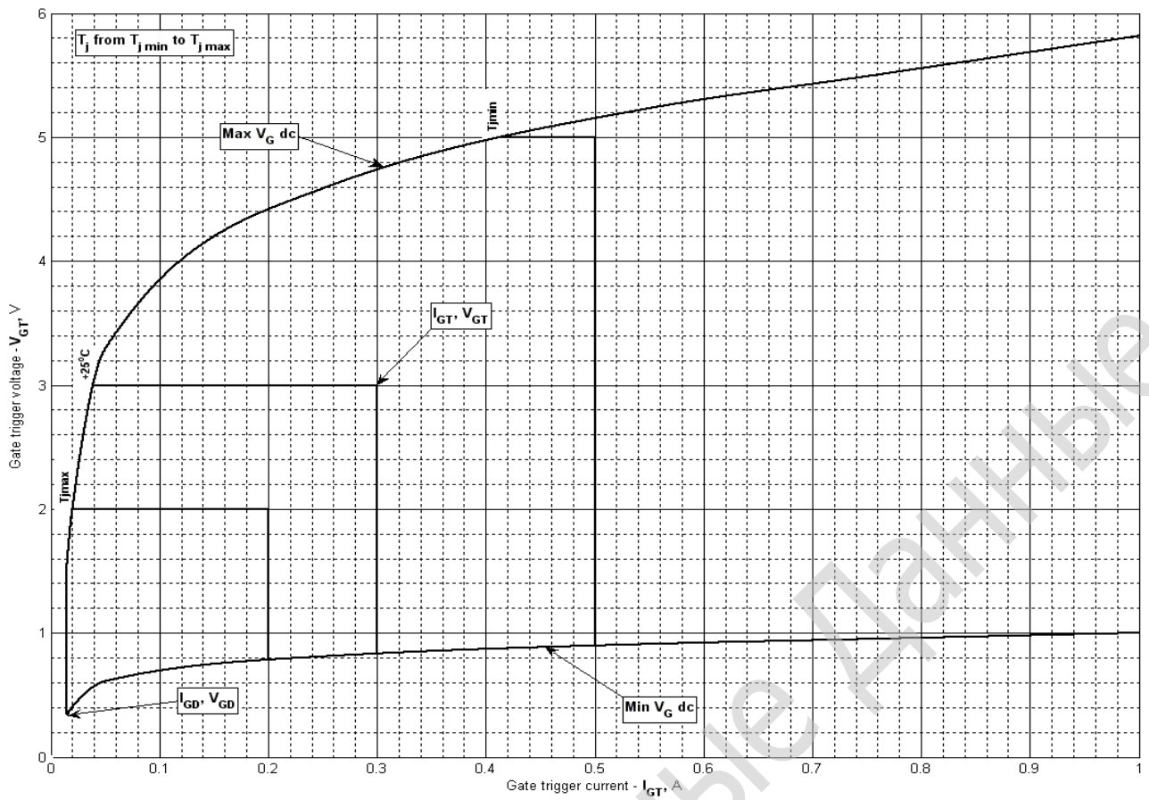
Рис. 3 – Вольт – амперная характеристика цепи управления
