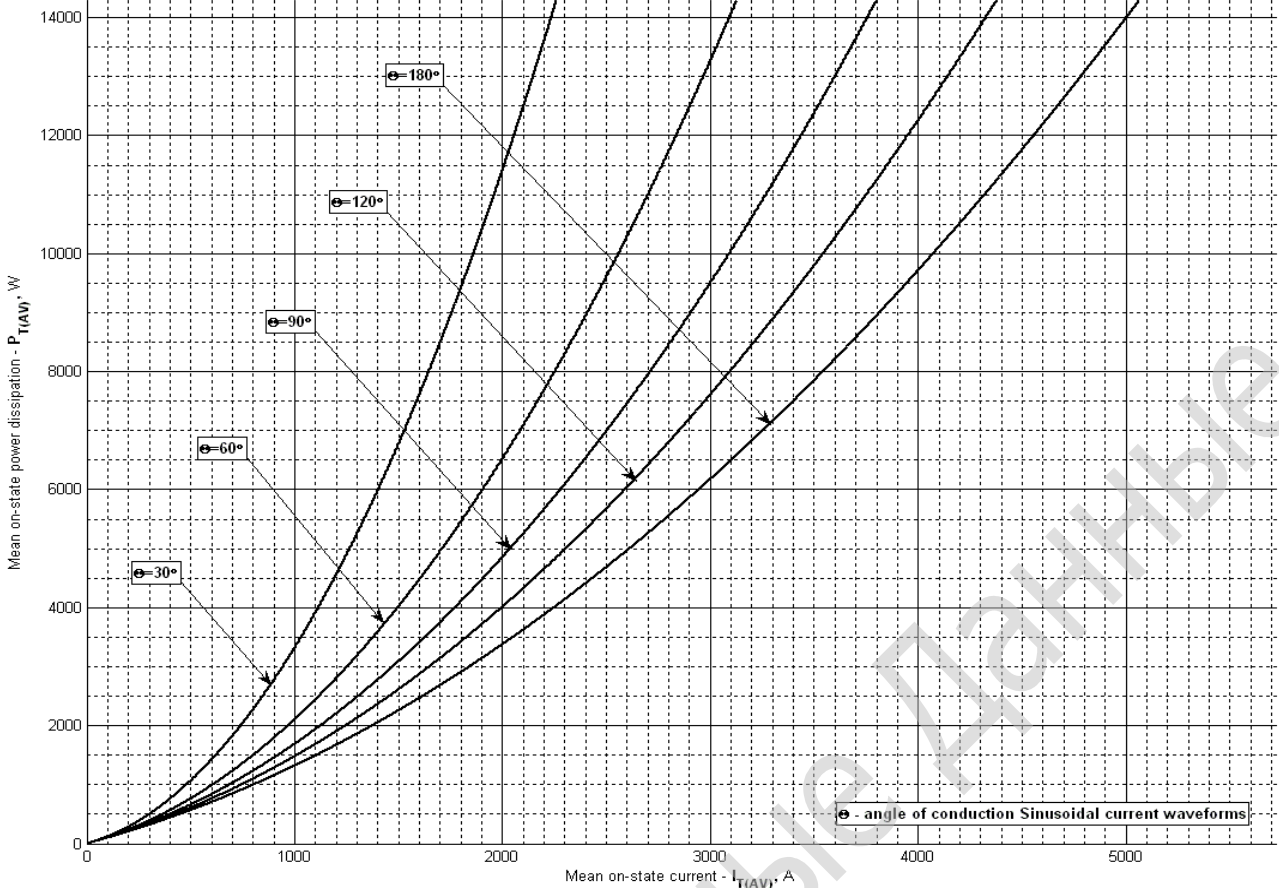
Рис. 9 - Зависимость потерь мощности P_{TAV} от среднего тока в открытом состоянии I_{TAV} синусоидальной формы при различных углах проводимости ( f=50 Гц, двухстороннее охлаждение)
