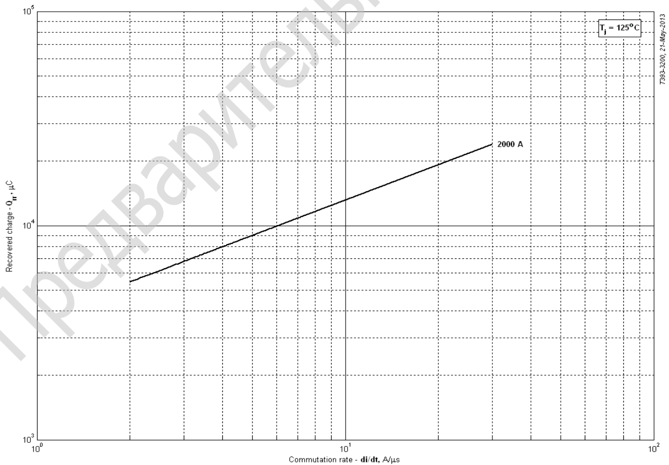
Рис. 6 – Зависимость максимального заряда обратного восстановления Q_{rr} от скорости спада тока di_R/dt (по ГОСТ 24461, хорда 25%) в открытом состоянии
