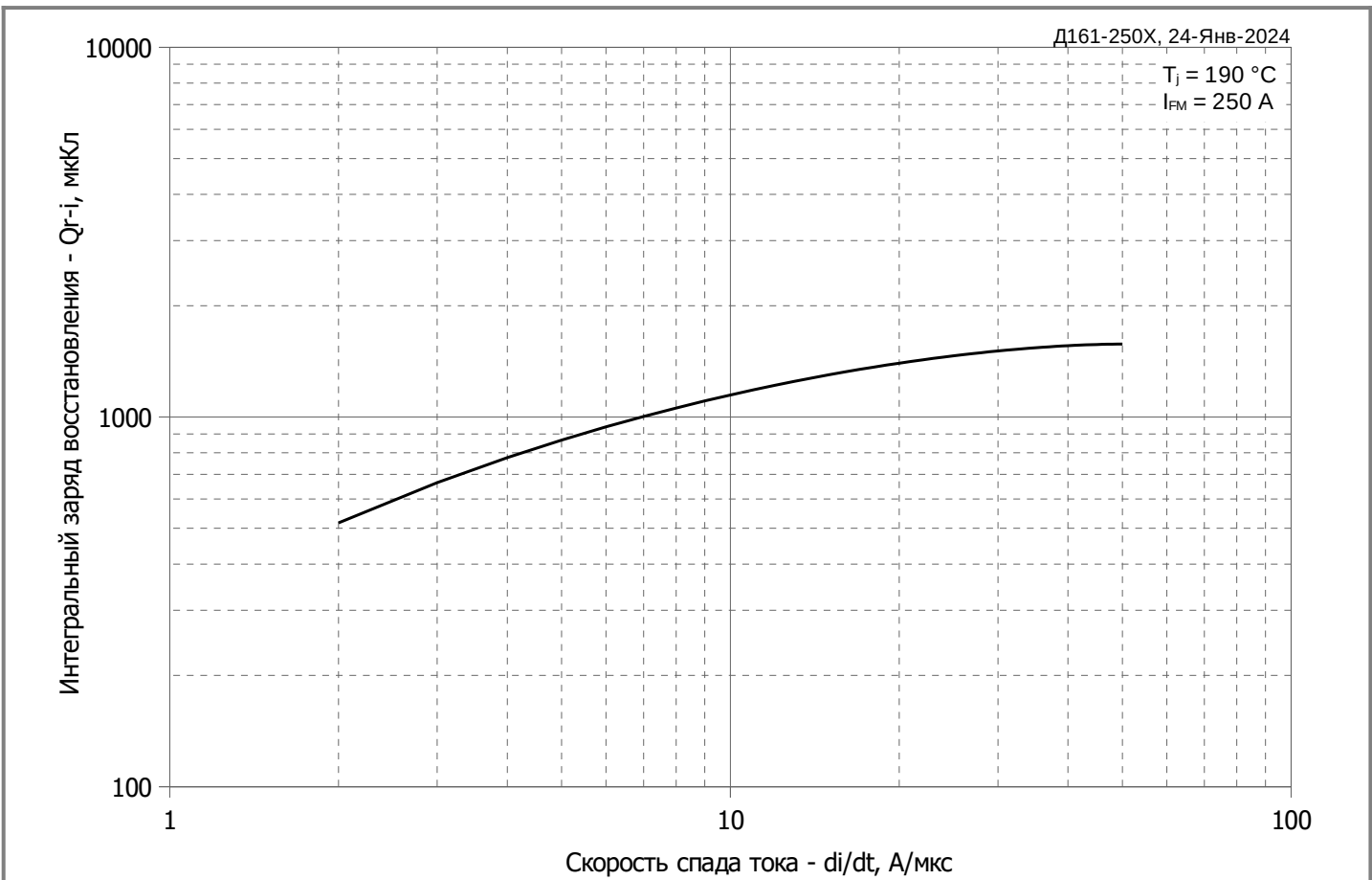
Рис. 3 – Зависимость максимального интегрального заряда обратного восстановления Q_{rr-i} от скорости спада прямого тока di_R/dt
