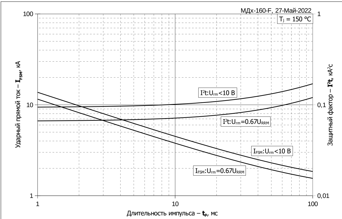
Рис. 11 – Зависимость максимальной амплитуды ударного прямого тока I_{\text{FSM}} и защитного фактора I^2t от длительности импульса t_p
