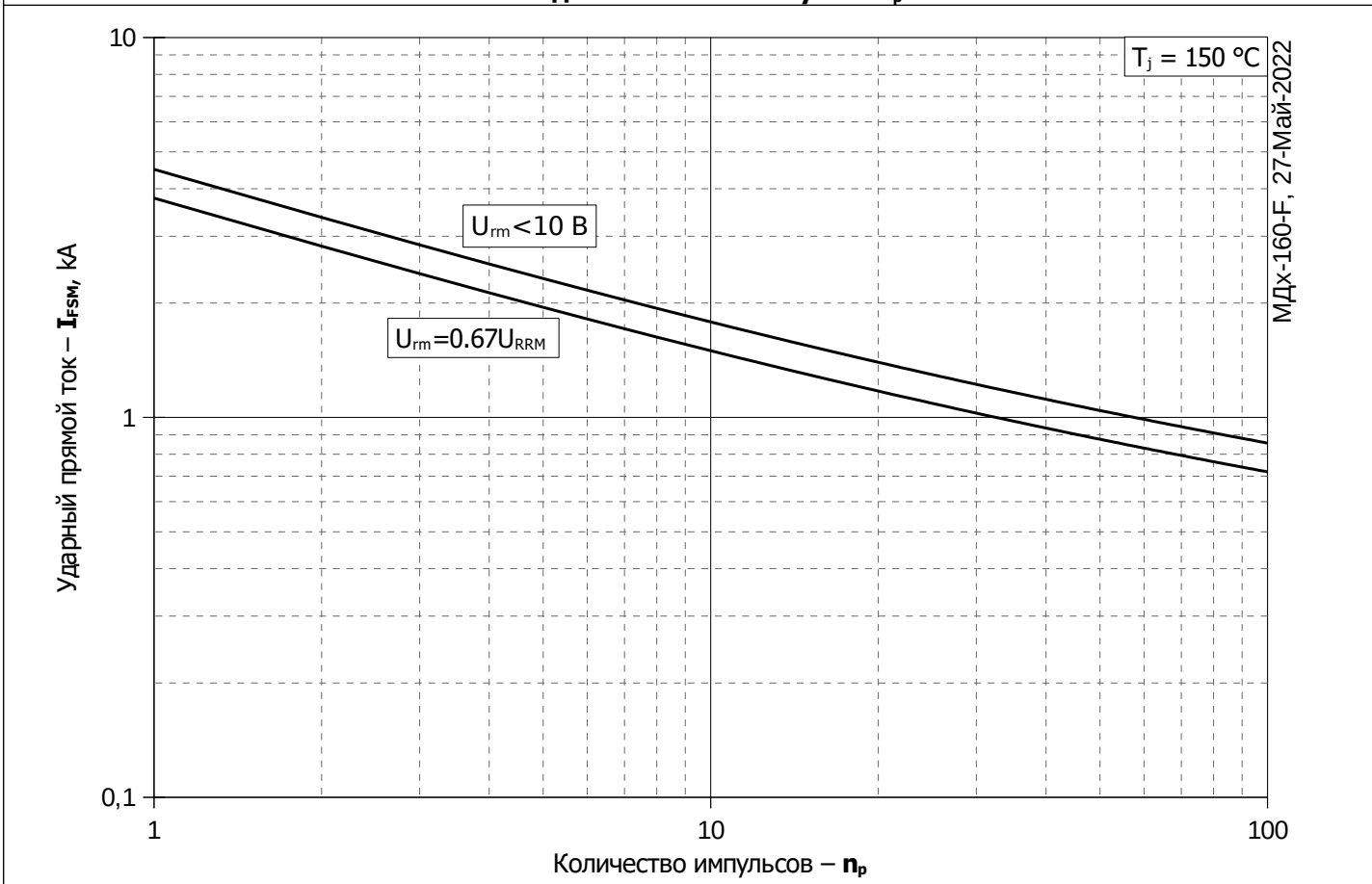
Рис. 12 – Зависимость максимальной амплитуды ударного прямого тока I_{\text{FSM}} от количества импульсов n_p
