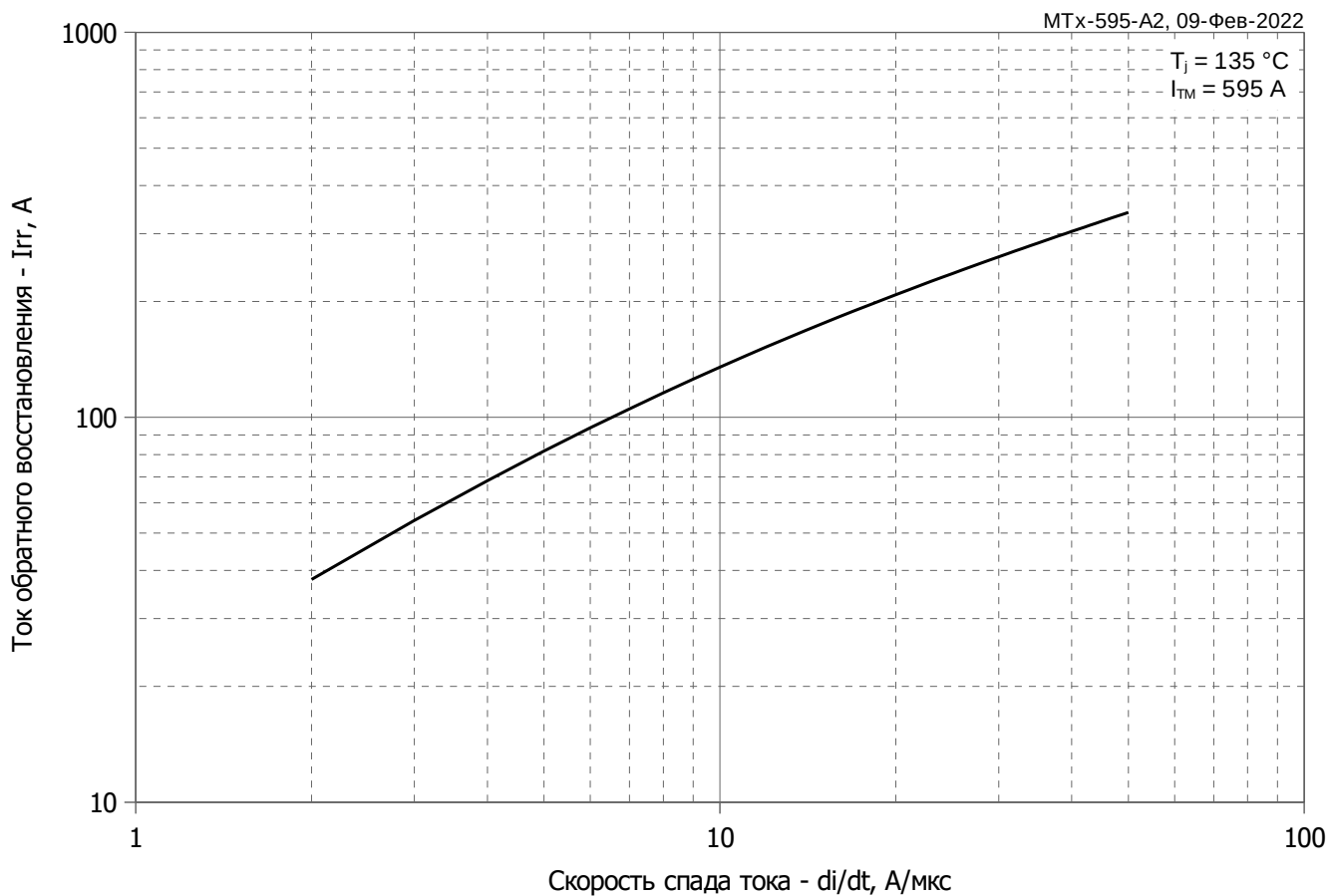
Рис. 7 – Зависимость максимального обратного тока восстановления I_{trr} от скорости спада тока di_R/dt в открытом состоянии
