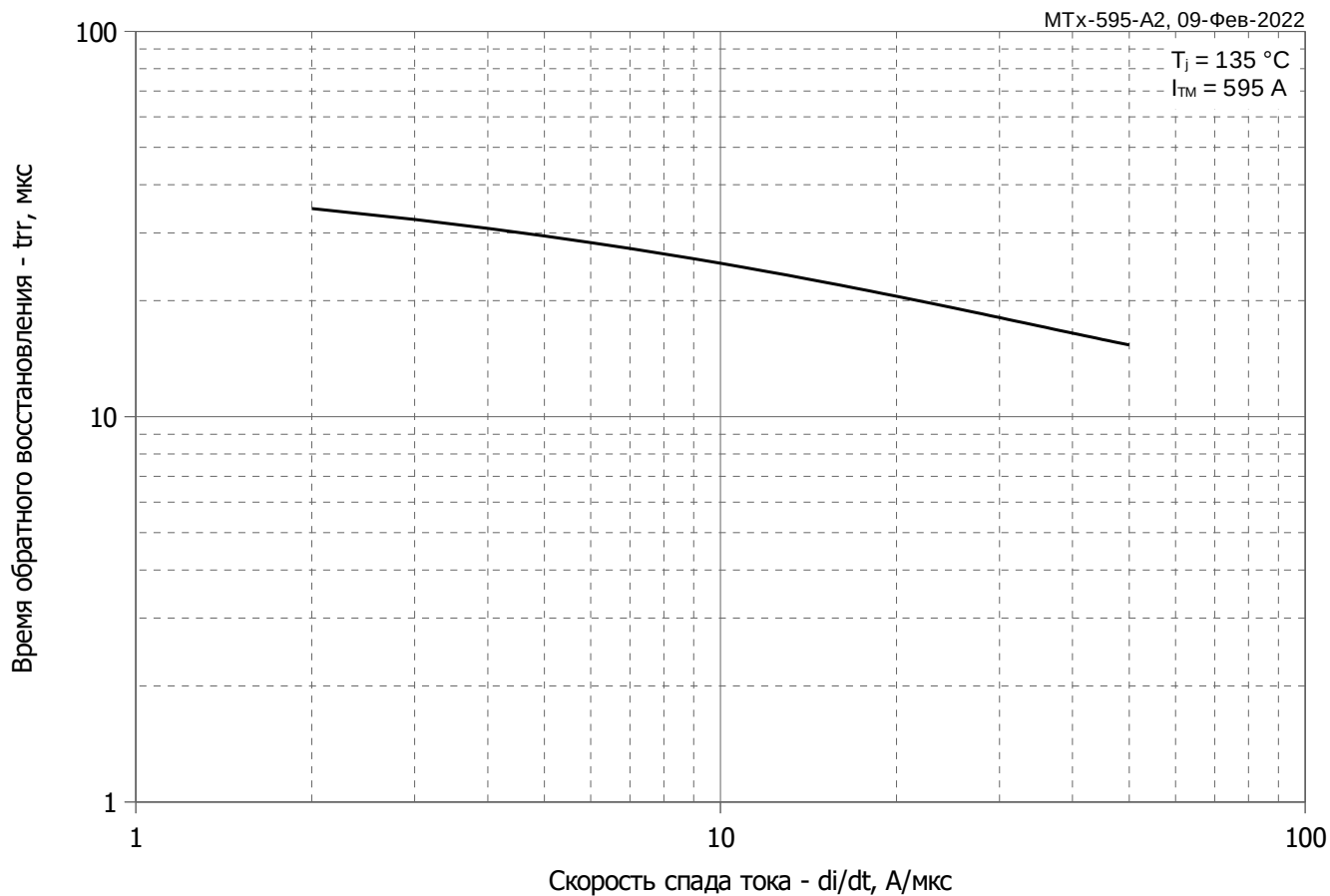
Рис. 8 - Зависимость максимального времени обратного восстановления t_{trr} от скорости спада тока di_R/dt (по ГОСТ 24461, хорда 25%) в открытом состоянии
