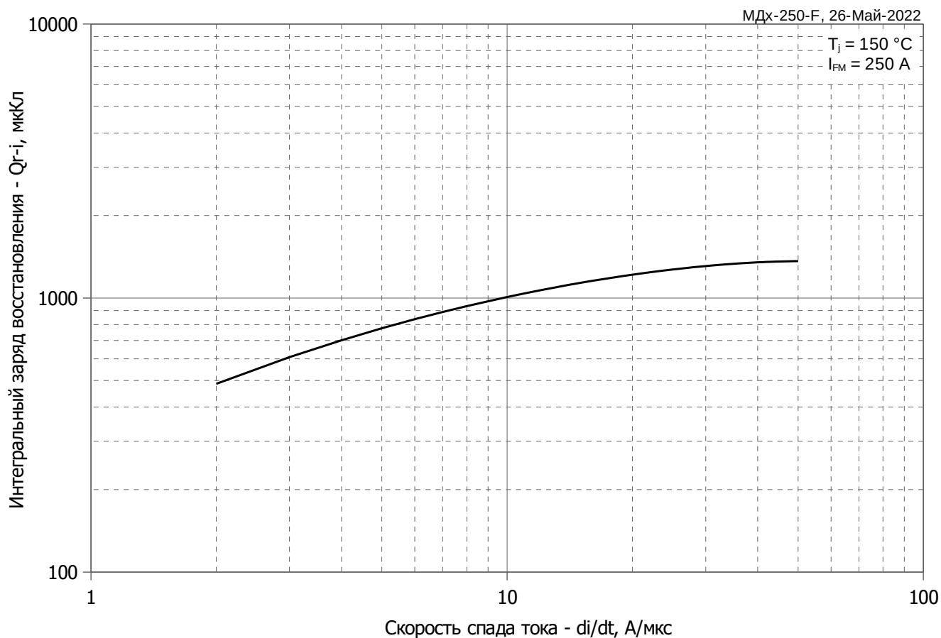
Рис. 3 – Зависимость максимального интегрального заряда восстановления Q_{g-i} от скорости спада прямого тока di_R/dt
