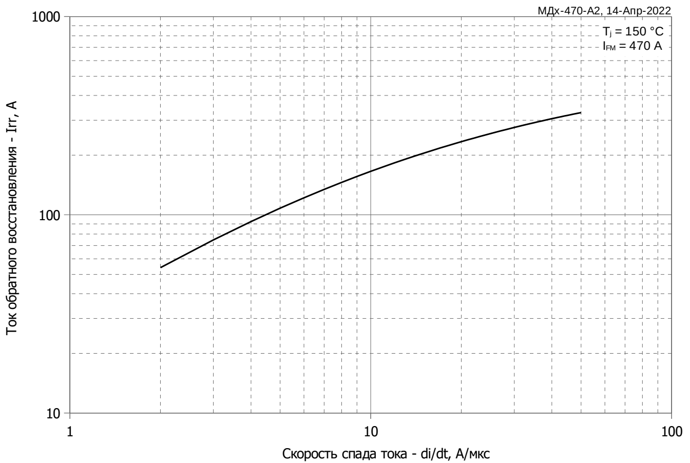
Рис. 5 – Зависимость максимального обратного тока восстановления I_{trr} от скорости спада прямого тока di_R/dt
