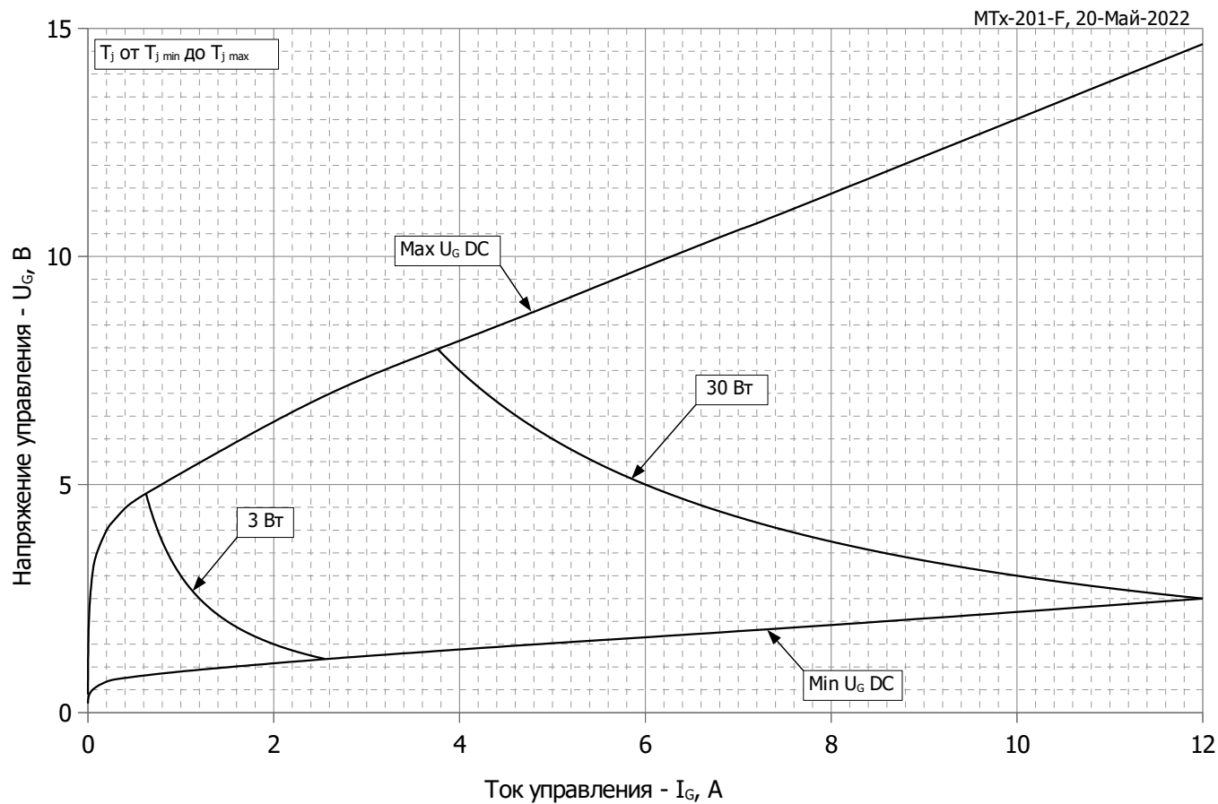
Рис. 3 – Вольт – амперная характеристика цепи управления — Кривые мощности
