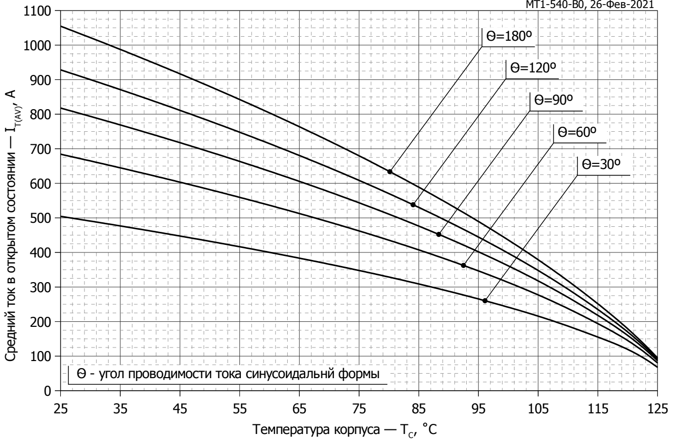
Рис. 8 – Зависимость среднего тока в открытом состоянии I_{TAV} от температуры корпуса T_c для синусоидальной формы тока при различных углах проводимости ( f=50 Гц, Двустороннее охлаждение)
