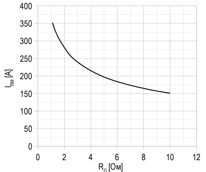
Рисунок 16 – типичная зависимость тока обратного восстановления от сопротивления в затворе, FRD.
