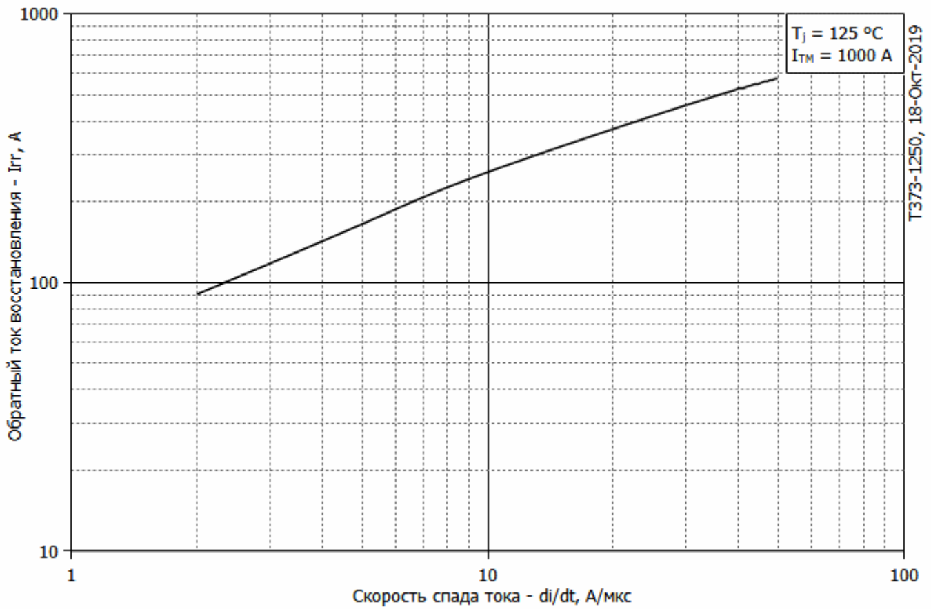
Рис. 5 – Зависимость максимального обратного тока восстановления I_{tr} от скорости спада тока di_R/dt в открытом состоянии
